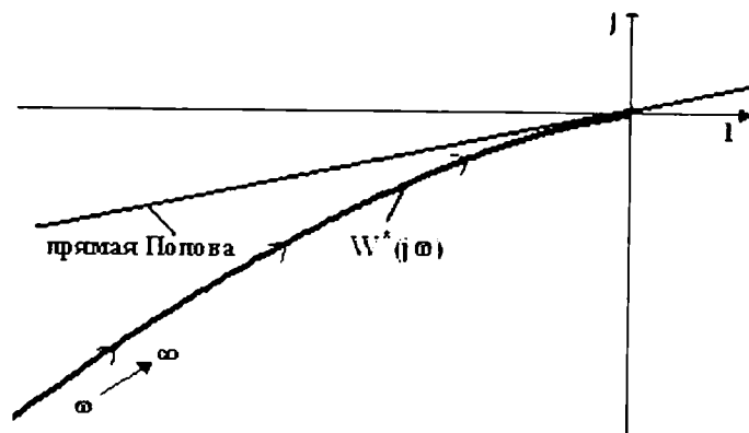
Рис. 7.4. Видоизмененная частотная характеристика.
