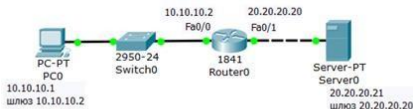
Рис. 9.17. Схема сети
