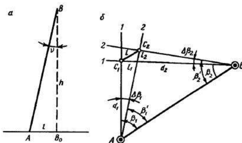
Рис. 1. Схемы определения крена сооружения: а - вертикальным проектированием, б - способом горизонтальных углов
