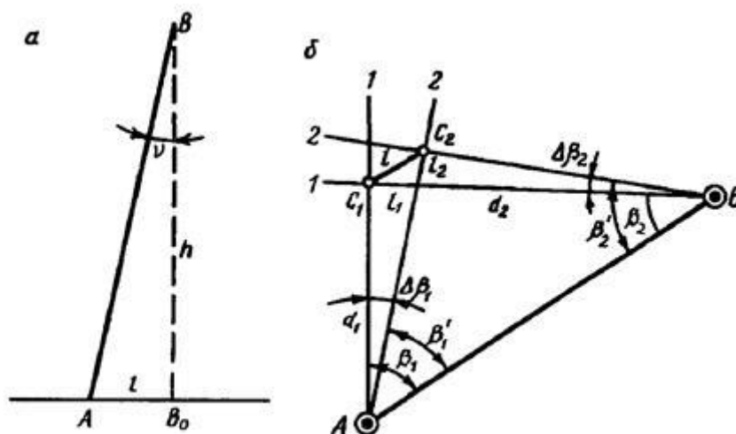
Рис. 1. Схемы определения крена сооружения: а - вертикальным проектированием, б - способом горизонтальных углов
