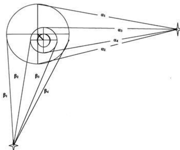
Рис. 2. Схема измерений горизонтальных углов при определении крена дымовой трубы в двух плоскостях близких к 90^{\circ}
