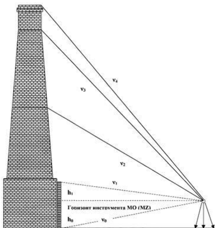
Рис. 3. Измерение горизонтальных углов на различных сечениях (зенитных расстояниях)
