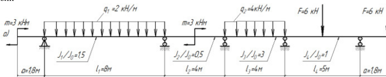
Рис.3. Расчётная схема балки
