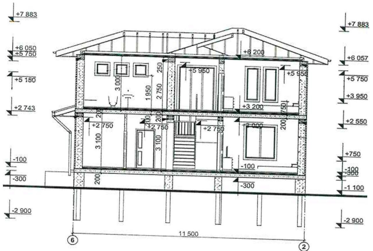
Рис.8 – Разрез 2-2
