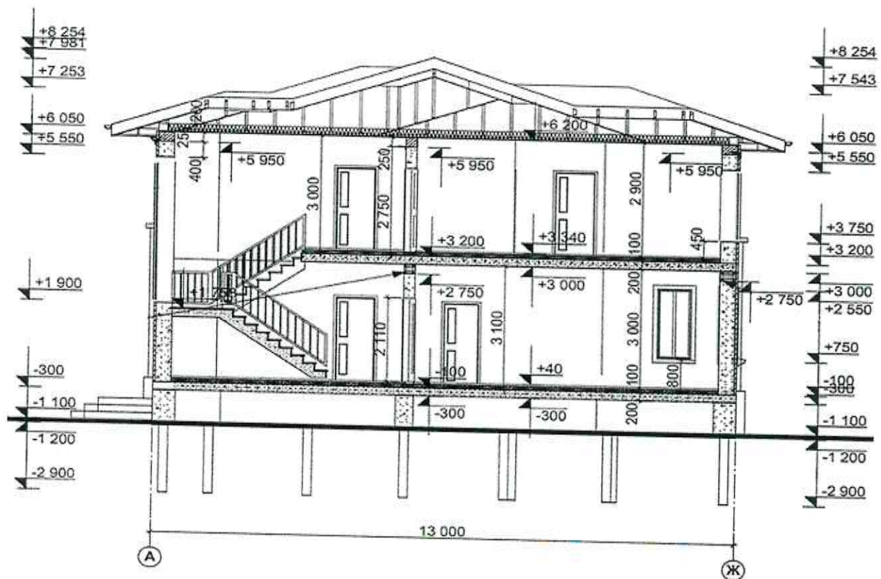
Рис.7 – Разрез 1-1
