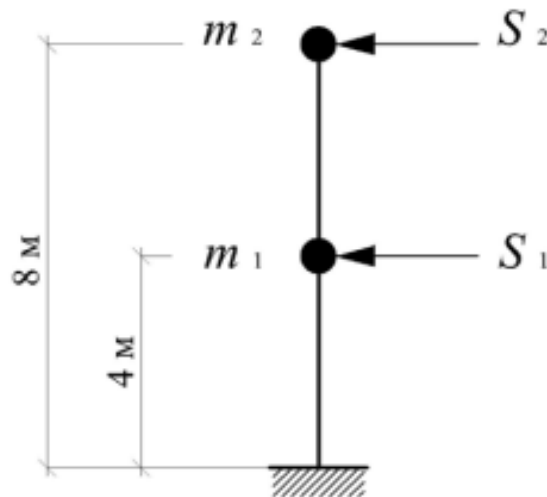
Рис.4.3. К примеру определения расчетной сейсмической нагрузки на здание
