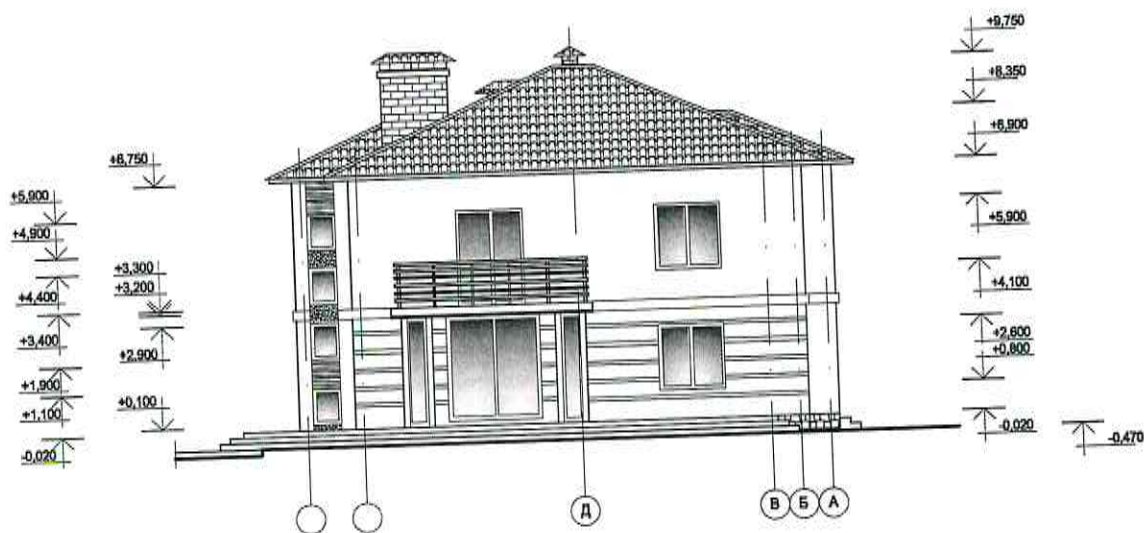
Фасад Ж ÷ А
