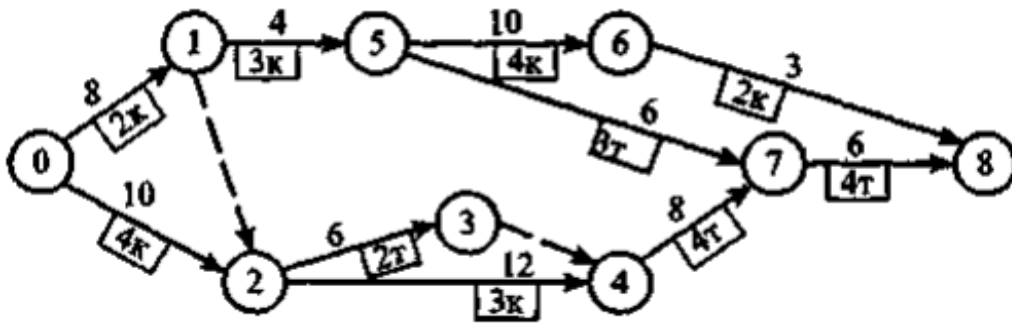
Рис. Сетевой график комплекса работ
