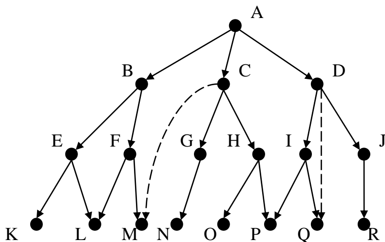
Рис.2 Граф состояний
