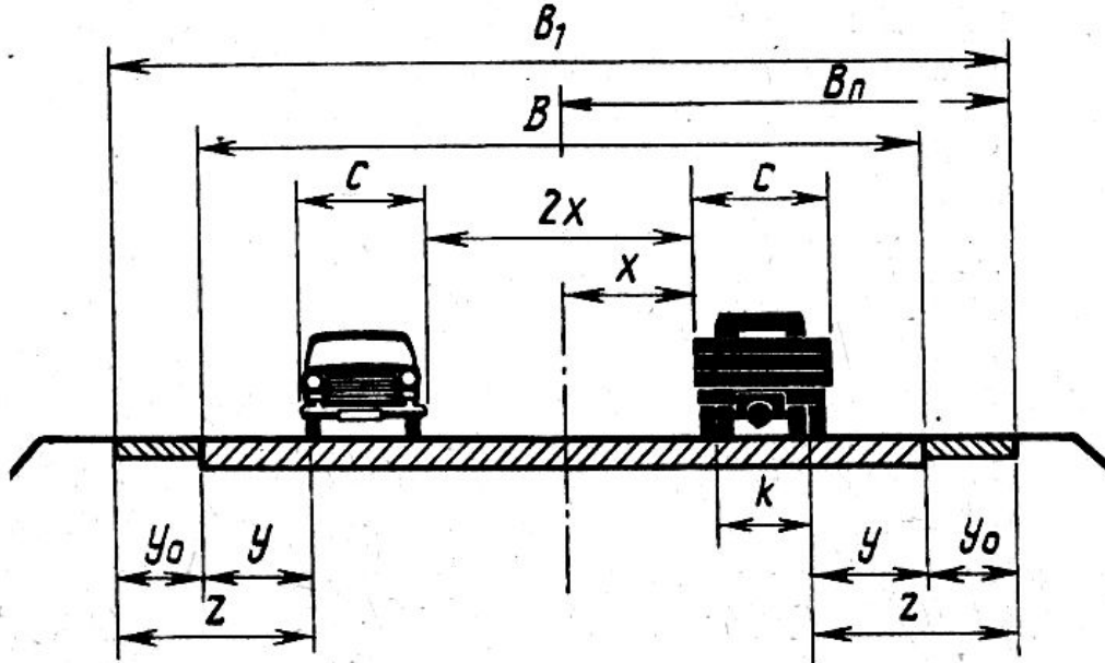
Рисунок 1 - Расчетная схема для определения ширины укрепленной поверхности при встречном движении
