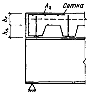
Рисунок 1.5 – Схема армирования торцовых частей монолитной плиты
