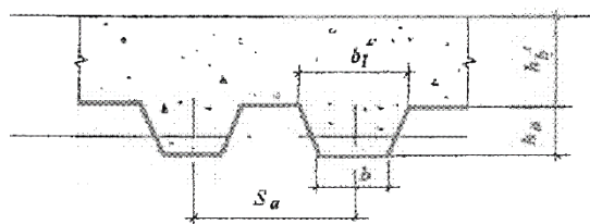
Рисунок 3 – Поперечное сечение плиты
