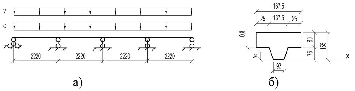
Рисунок 1.4 – Расчетная схема монолитного перекрытия (а) и расчетное тавровое сечение (б)
