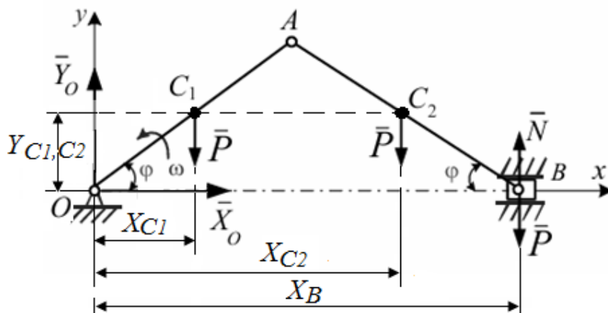
Рис.3.6. Расчетная схема
