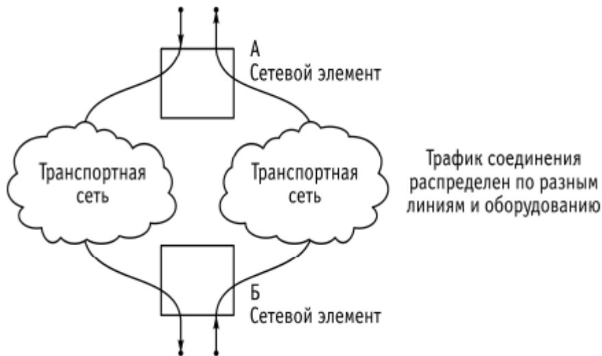
Рисунок 2в – Пример двунаправленного соединения с раздельной передачей
