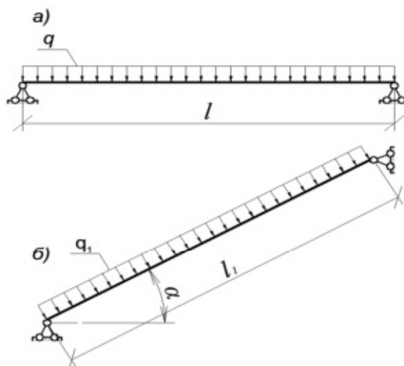
а)- Расчетная схема бруса. б)- Расчетная схема стропила.
