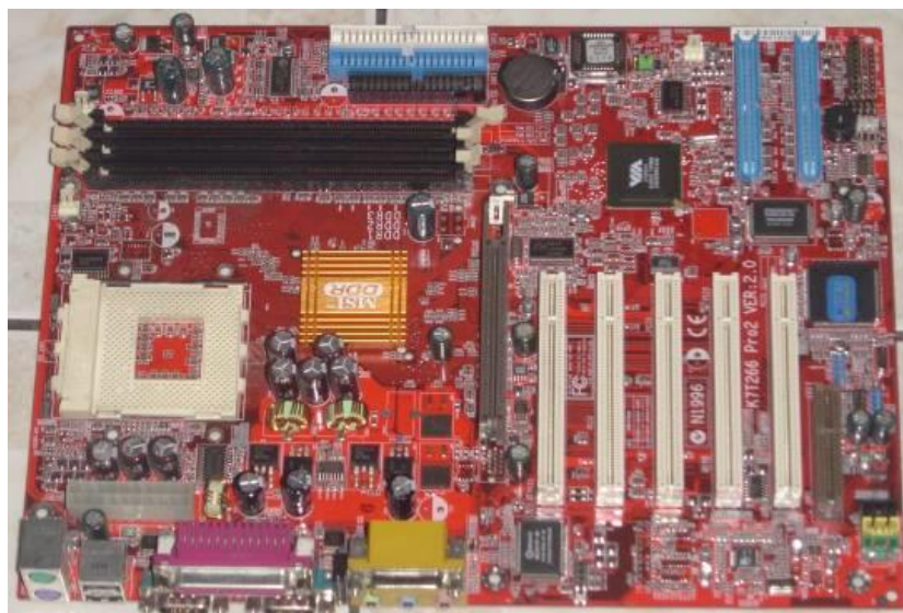
Рисунок 3 - Материнская плата стандарта ATX персонального компьютера (пример)
