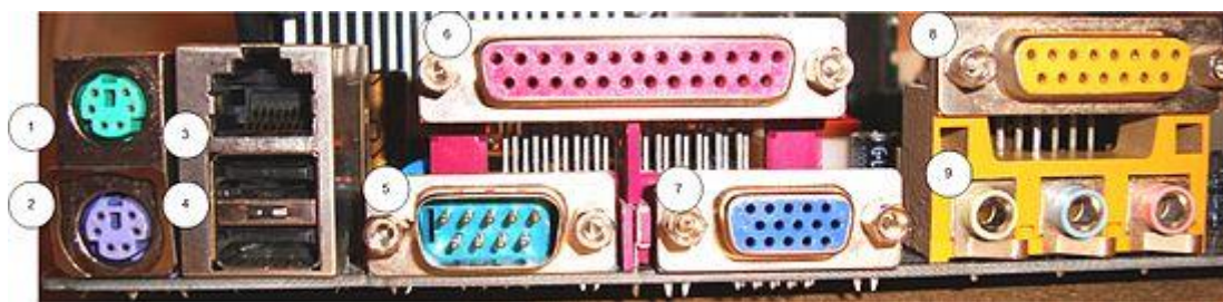
Рисунок 2 - Наружные разъемы материнской платы формата АТХ (пример)
