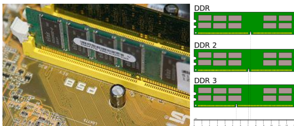
Рисунок 8 - Ключ-выемка на модуле и защёлки на разъёме препятствуют некорректной установке модуля памяти
