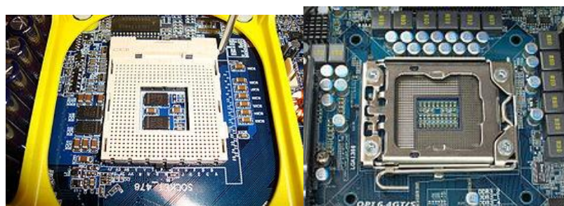
Рисунок 4 - Разъёмы центрального процессора Intel: Socket 478 (процессоры Pentium 4, Celeron) и LGA 1366 (процессоры Core i7, Xeon) (пример)
