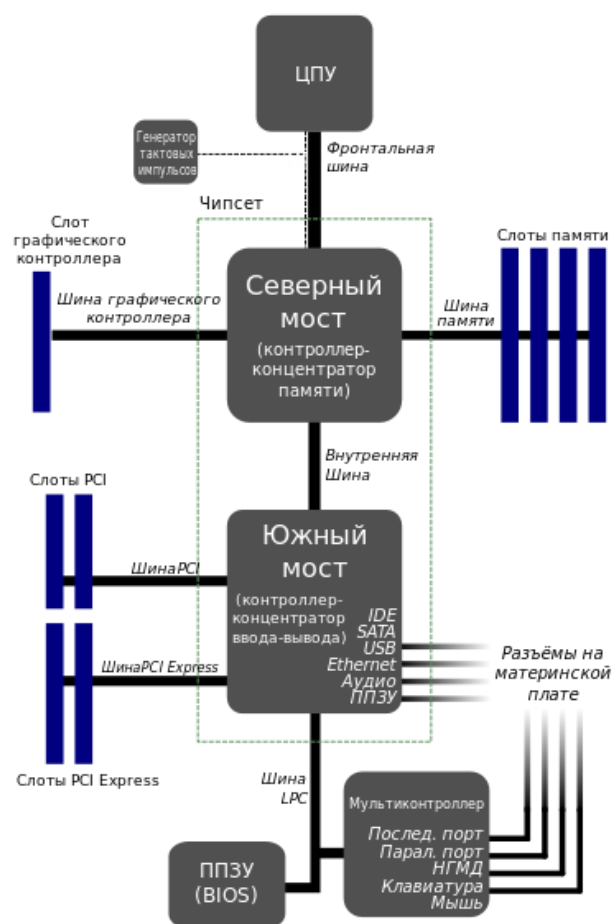
Рисунок 5 - Схематическое изображение традиционного чипсета материнской платы
