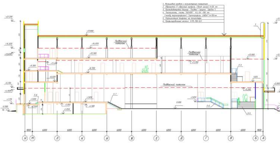
Разрез 2-2
