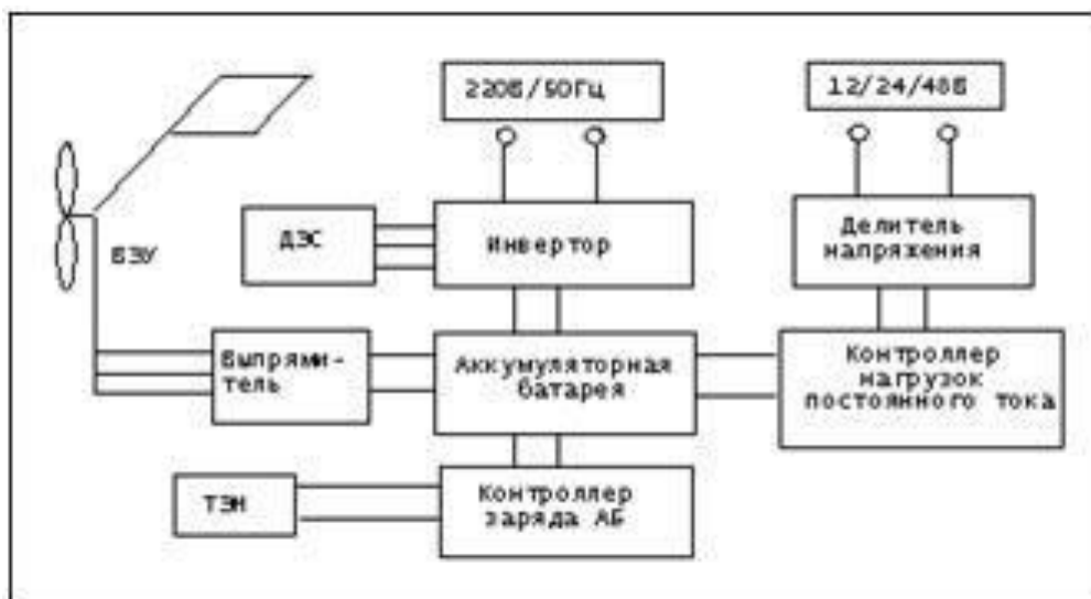
Рисунок 5 - Структурная схема энергоустановки с использованием ВЭУ
