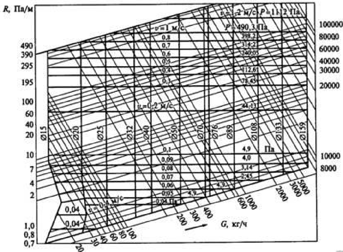
Рисунок 4.1 - Номограмма для расчета диаметров трубопроводов систем отопления при температуре воды 95... 70 °С
