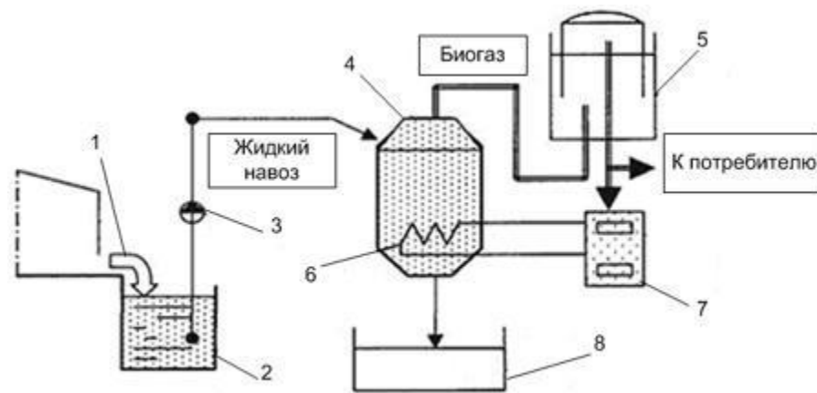
Рисунок 8 - Технологическая схема получения биогаза
