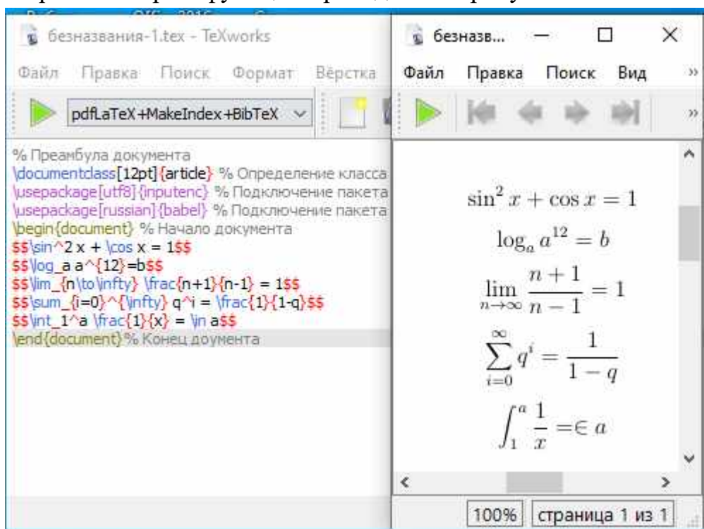
Рисунок 4 – Тригонометрические функции
