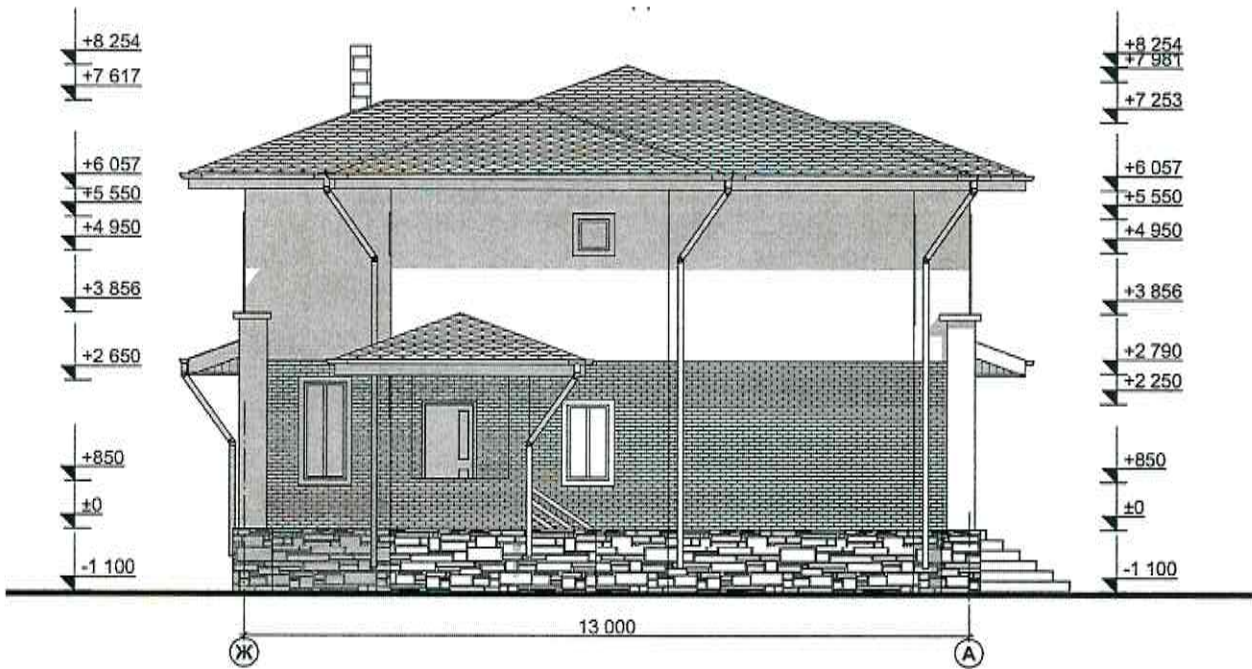
Рис.4 – Фасад Ж-А
