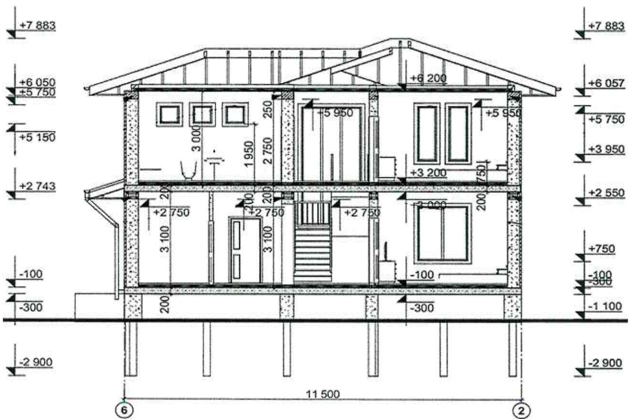
Рис.8 – Разрез 2-2
