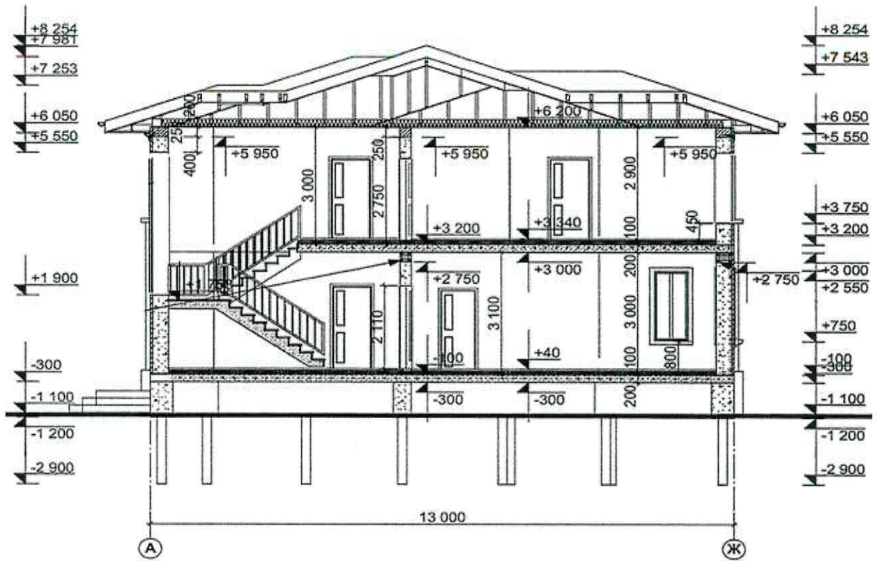
Рис.7 – Разрез 1-1
