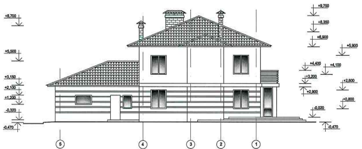
Фасад 5 ÷ 1
