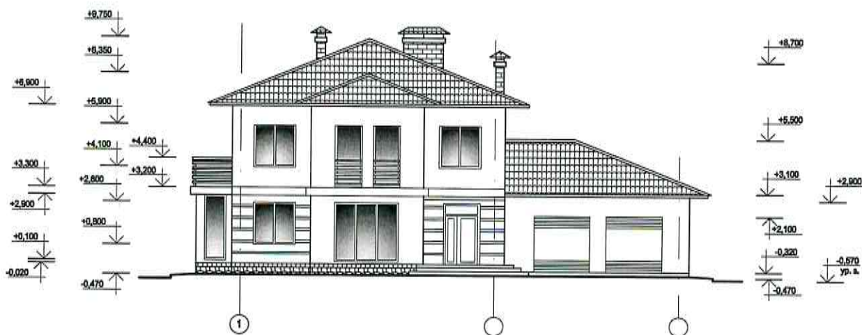
Фасад 1 ÷ 5
