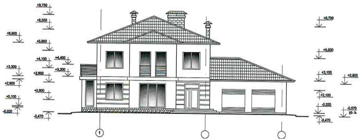
Фасад 1 ÷ 5
