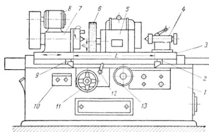
Круглошлифовальный станок
