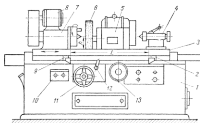
Круглошлифовальный станок
