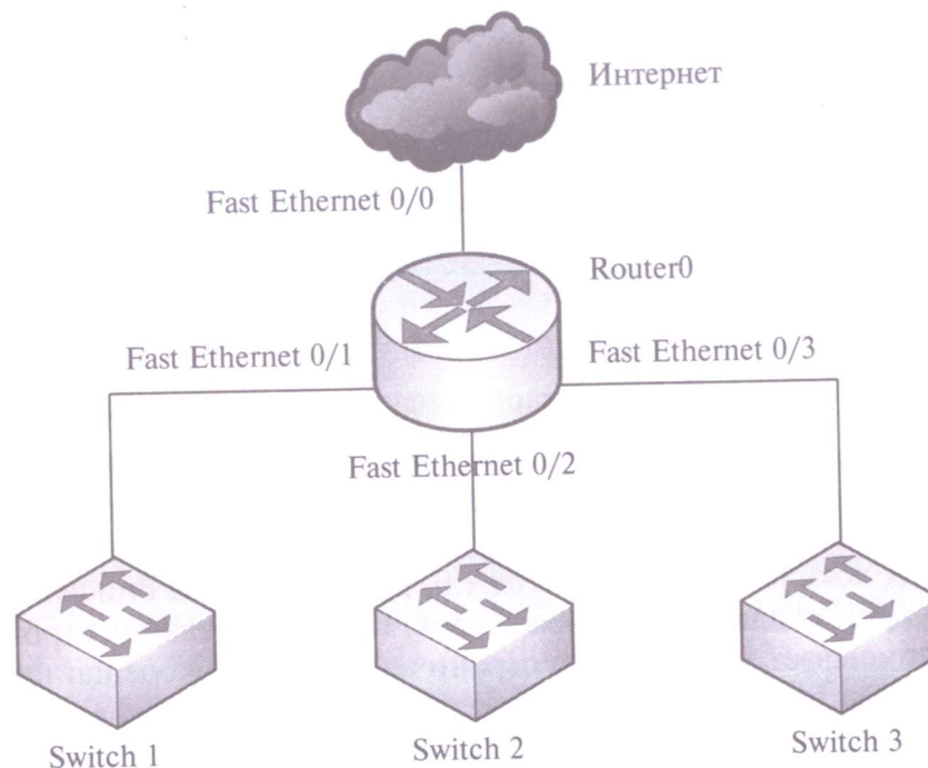
Рисунок 5.1 – Структура сети
