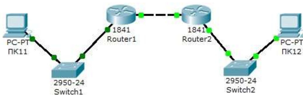
Рисунок 6.2 – Схема сети, где Switch1 – сеть 10.11.0.0/16, Switch2 – сеть 10.12.0.0/16, сеть для маршрутизаторов - 10.10.0.0/16
