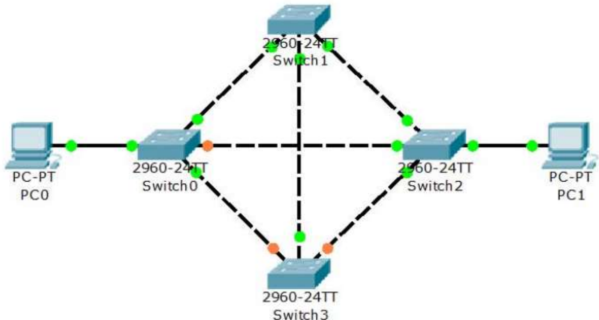
Рисунок 3.1 – Схема сети с избыточными линиями связи
