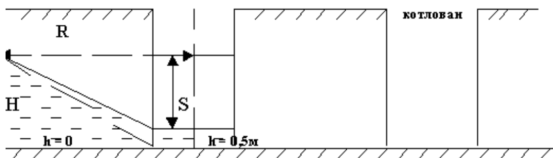
Рис. 5. Перехват потока грунтовых вод канавой
