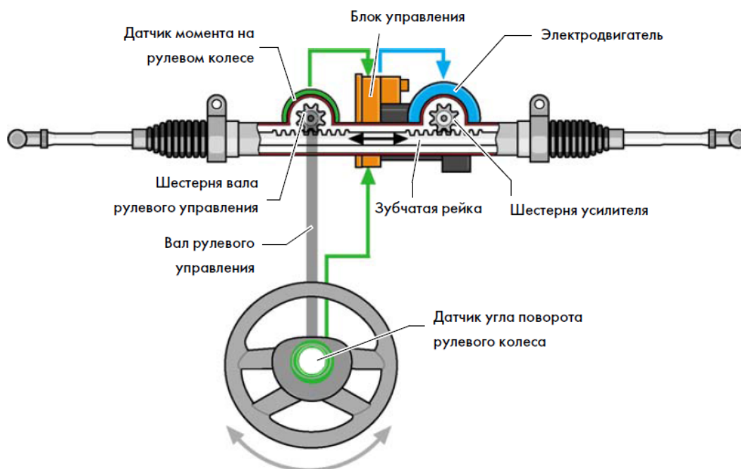
Рис. 1.1 Электромеханический усилитель руля
