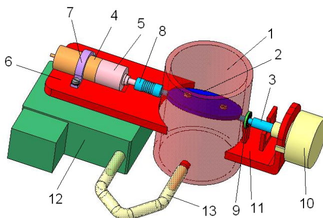
Рис. 1.6 Однодрельная система:
