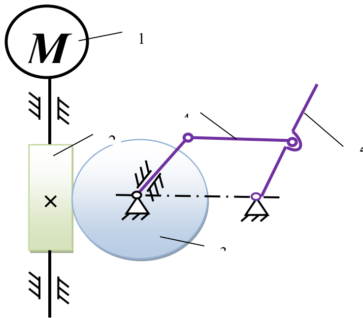
Рис. 1.9 Привод автоматической распашной двери:
