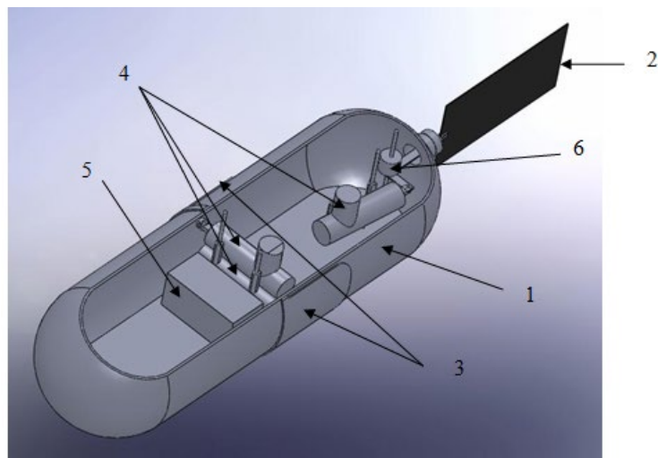
Рис. 1.3 Робот-рыба:
