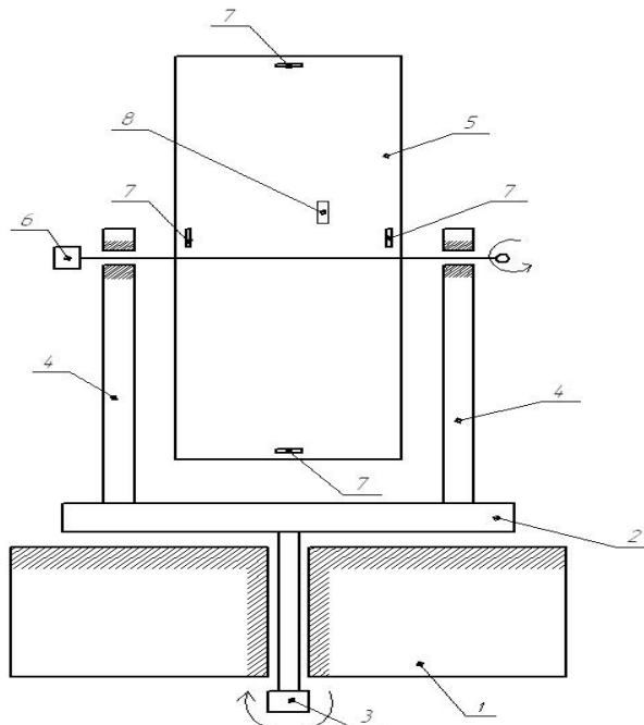
Рис. 1.10 Схема автоматической солнечной установки:
