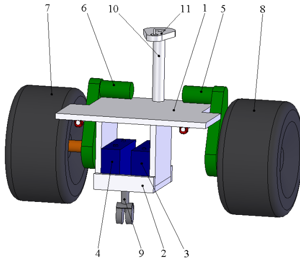
Рис. 1.2 Колесная платформа для мониторинга местности:
