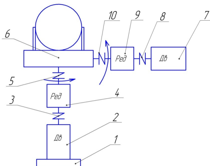
Рис. 1.8 Устройство наведения антенны: 1 – основание, 2, 7 – двигатели, 4, 9 – редукторы, 3, 5, 8, 10 – муфты, 6 – антенна
