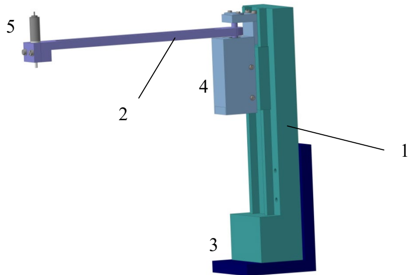
Рис. 1.3 Манипулятор для завинчивания пробок:
