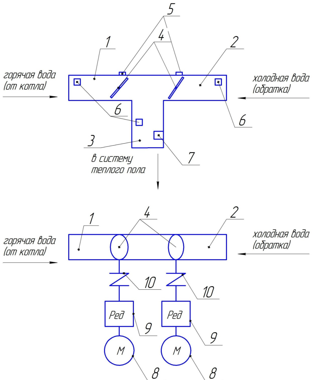
Рис. 1.9 Система теплого пола:
