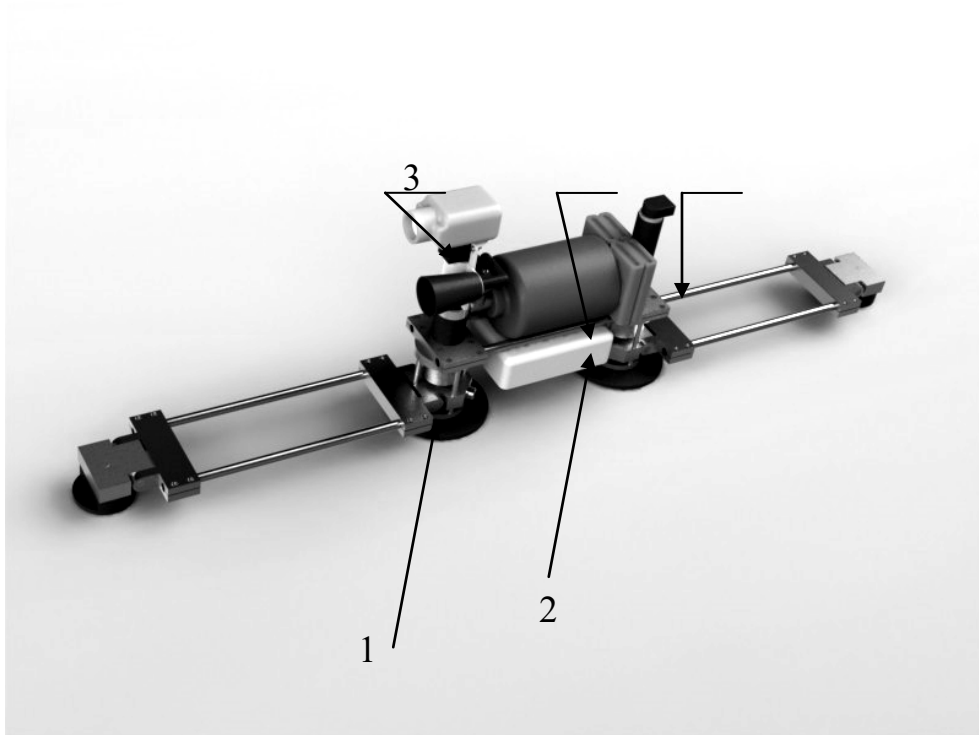
Рис. 1.4 Ползающий трехзвенный робот-пожарник:
