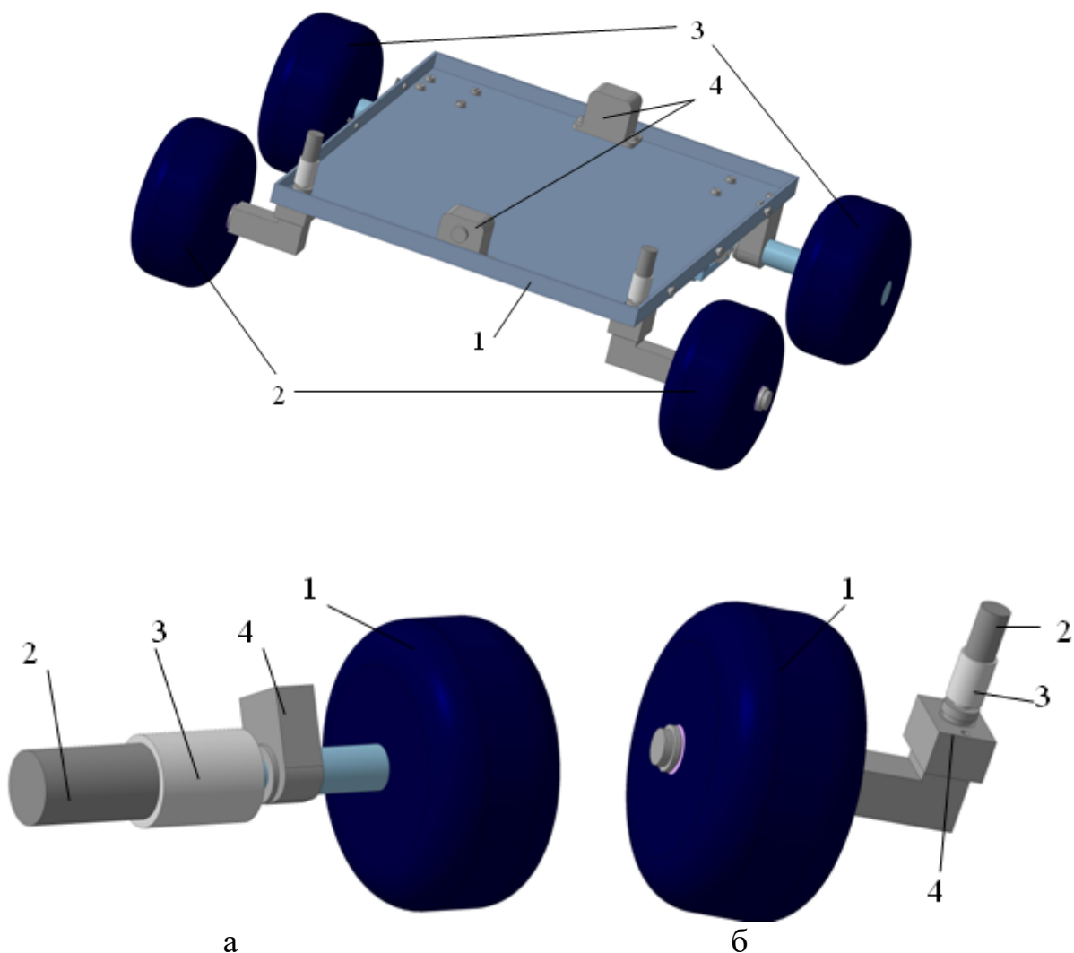
Рис. 1.4 Телеуправляемый колесный робот (кожух не показан):
