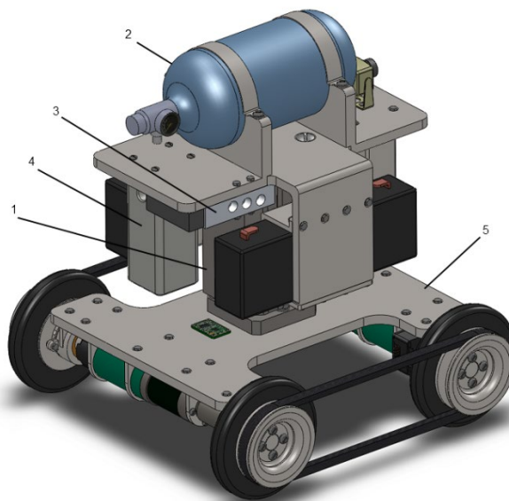
Рис. 1.7 Прыгающий робот:
