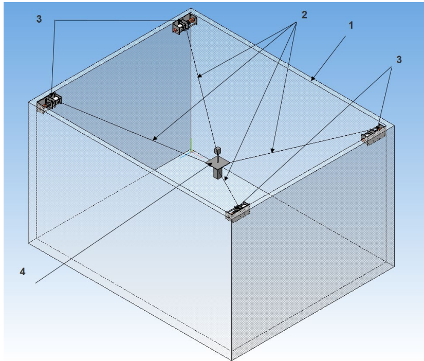
Рис. 1.2 Устройство позиционирования видеокамеры на стадионе: 1- основание, 2 – синтетические тросы, 3 – электролебедки,
