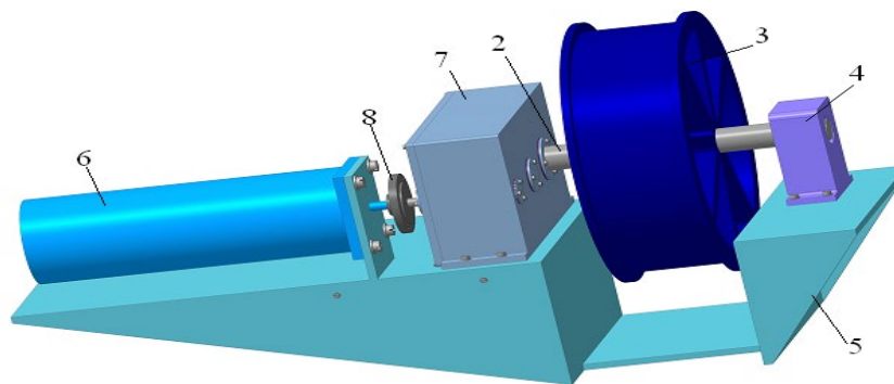
Рис. 1.5 Привод вращательного движения:
