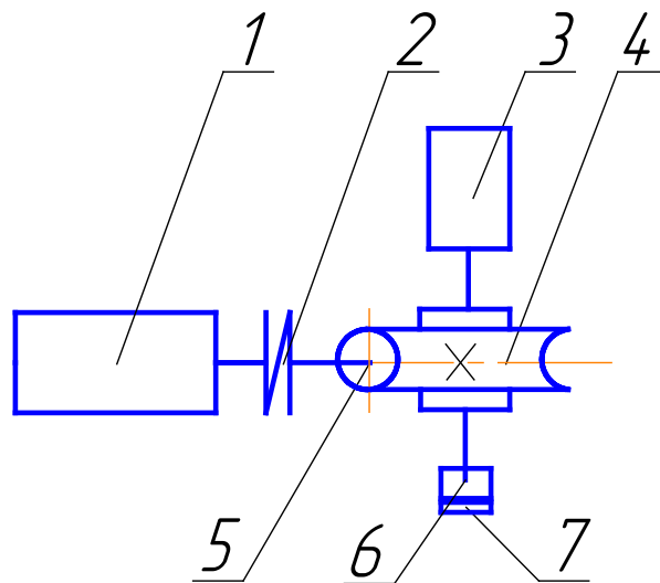
Рис. 1.10 Поворотное устройство видеокамеры:
