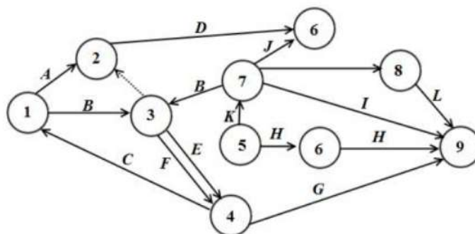
Рисунок – Сетевая модель для выполнения задания
