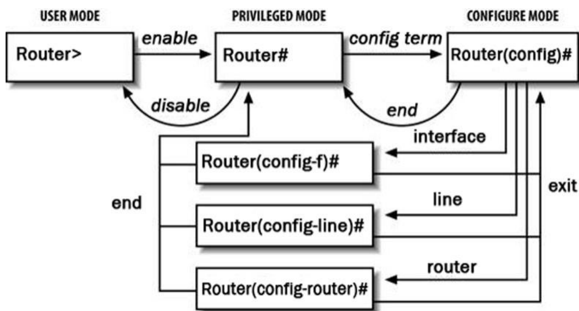
Рисунок 13 - Схема контекстов Cisco IOS (пример для маршрутизатора)
