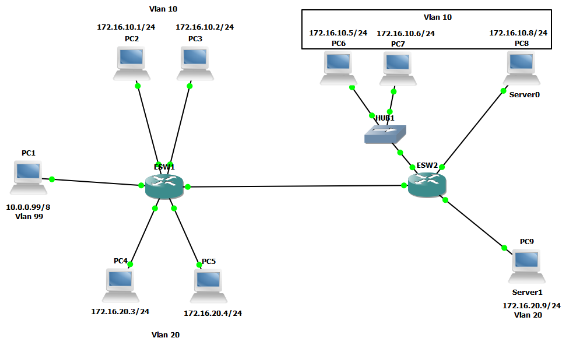
Рисунок 3 - Схема сети с магистральным каналом
