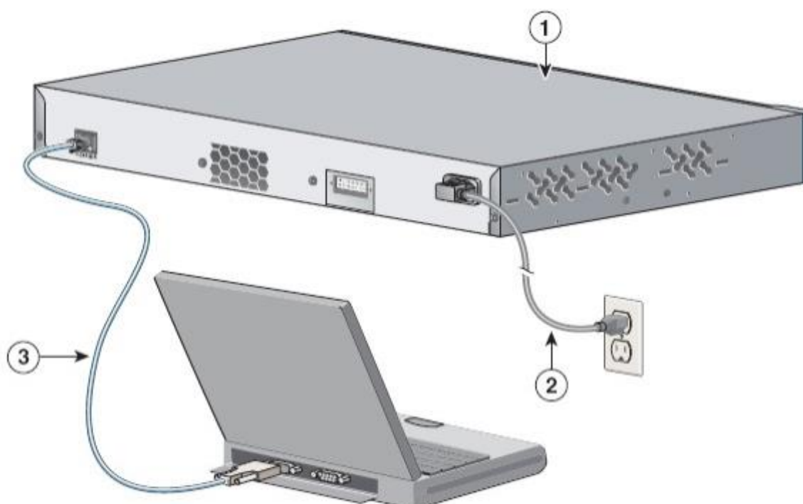
Рисунок - 11 Подключение по консольному кабелю
