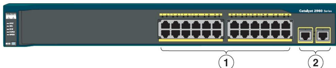
Рисунок - 10 Лицевая панель Catalyst 2960-24TT (1 – 10/100 порты; 2 – 10/100/1000 порты)
