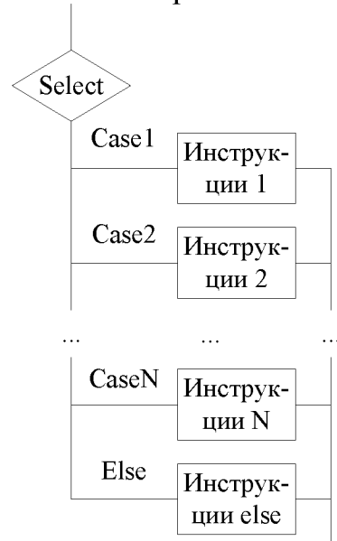
Схема алгоритма оператора Select Case
