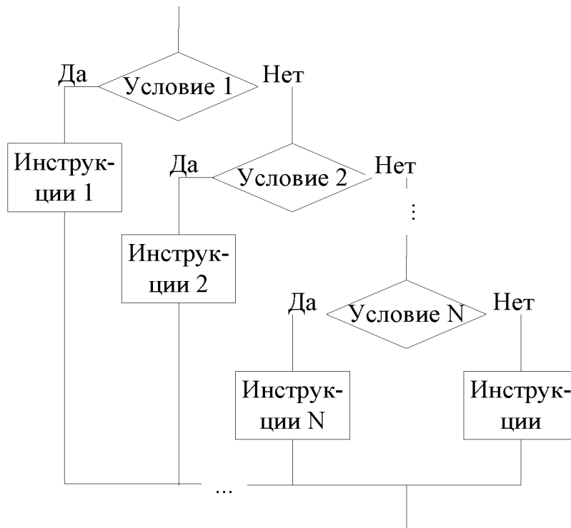
Схема алгоритма оператора If Then ElseIf .
