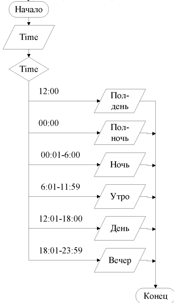
Схема алгоритма программы определения времени суток
