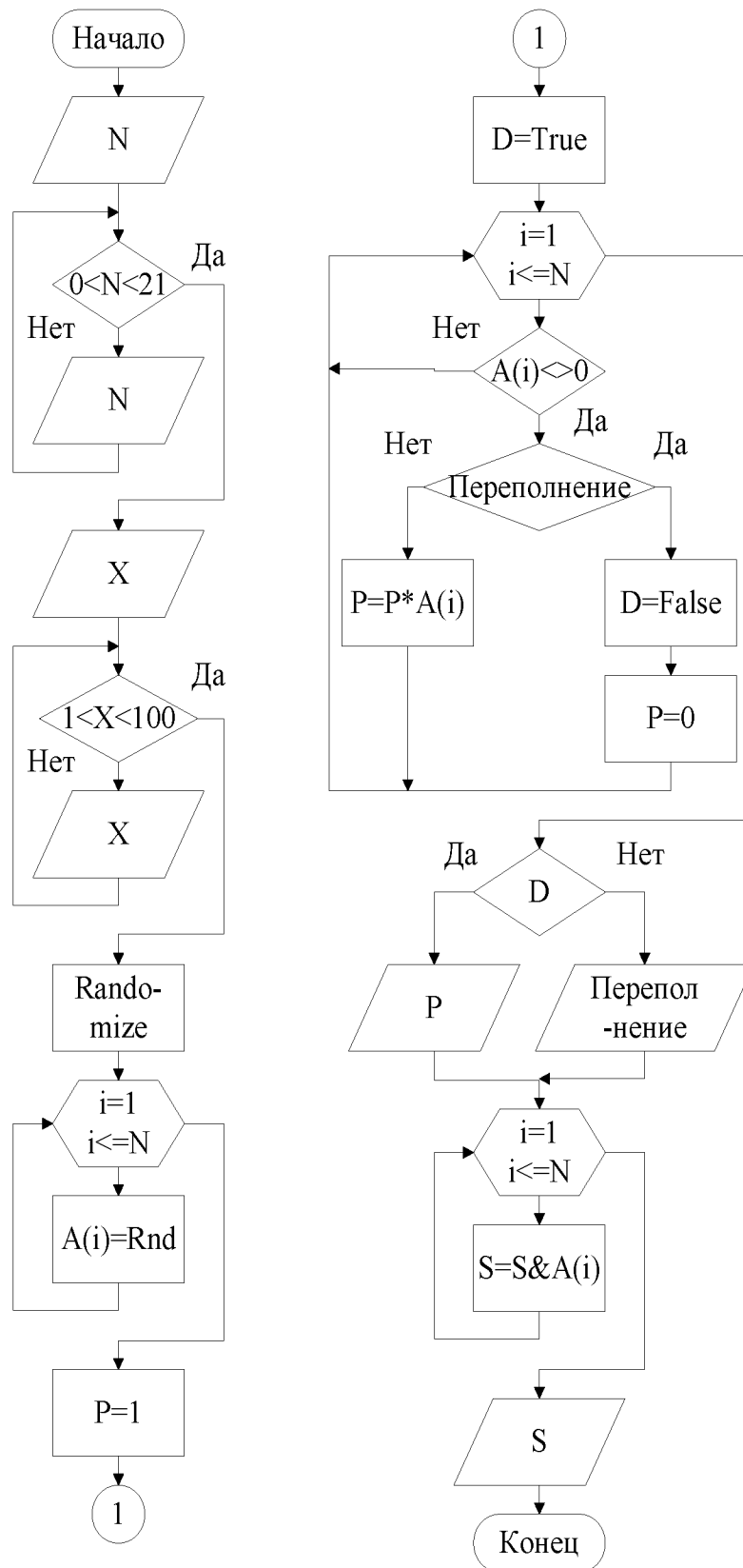
Алгоритм программы вычисления произведения ненулевых элементов массива.
