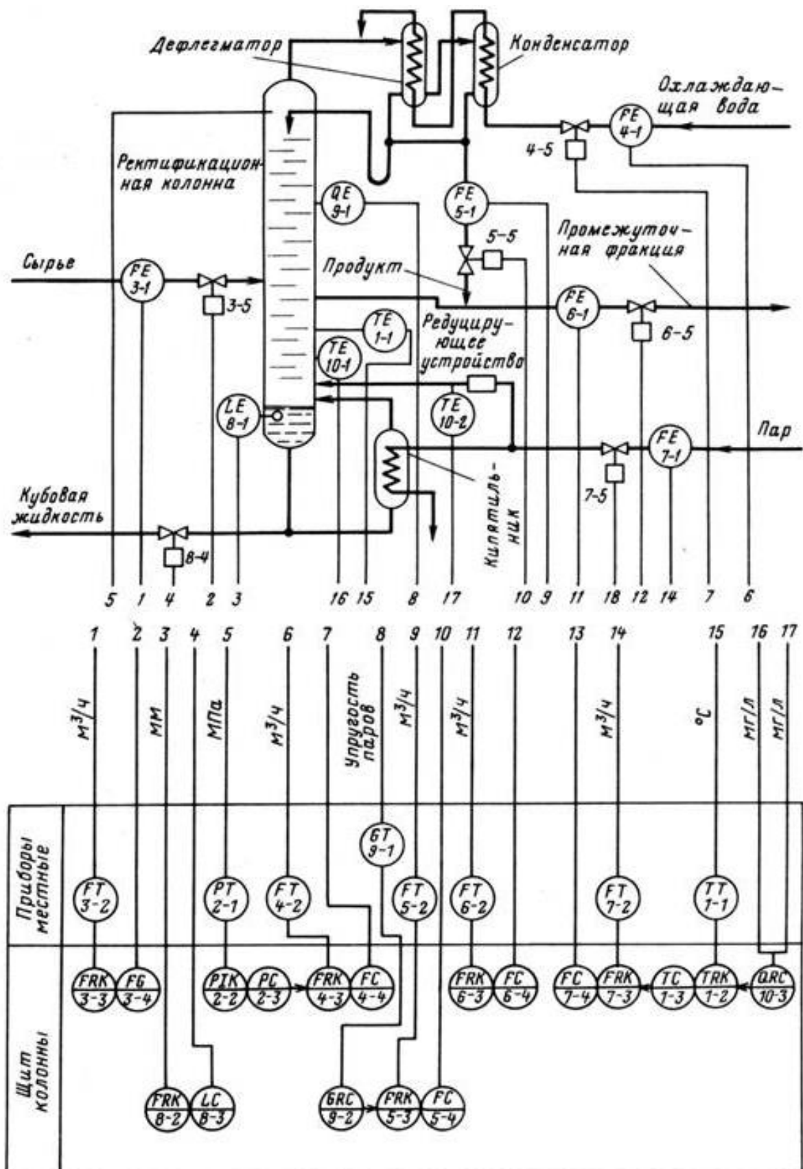
Рисунок 2 – Пример выполнения функциональной схемы автоматизации по первому способу с изображением приборов по ГОСТ 21.404-85
