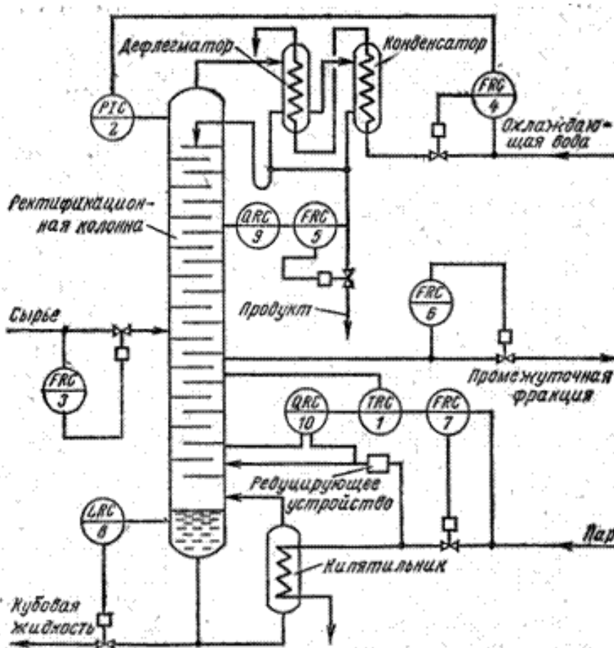
Рисунок 3 – Пример выполнения функциональной схемы автоматизации по второму способу
