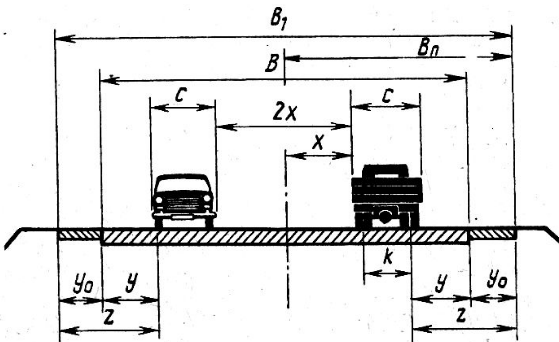
Рисунок 4 - Расчетная схема для определения ширины укрепленной поверхности при встречном движении:
