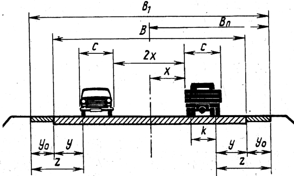
B_1 – ширина укрепленной поверхности; B_{\Pi} – ширина психологического коридора. Рисунок 1 - Расчетная схема для определения ширины укрепленной поверхности при встречном движении
