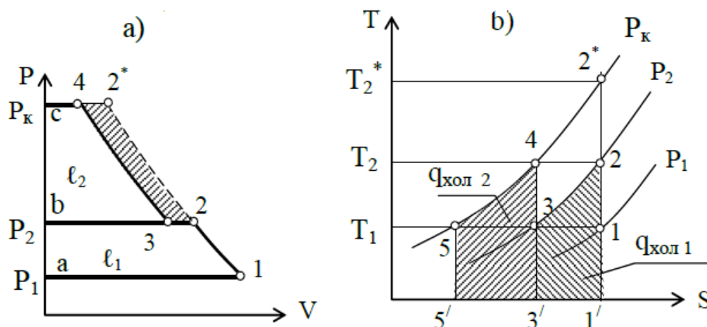
Рис.3 Процессы сжатия газа в двухступенчатом компрессоре
