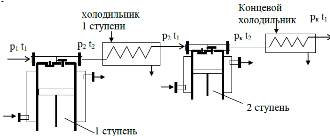
Рис.2. Схема 2-х ступенчатого компрессора
