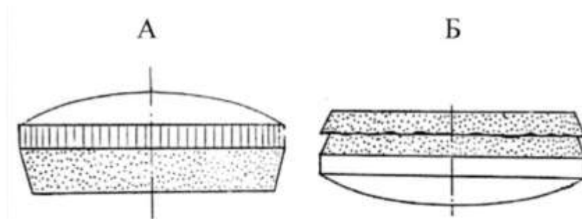
Рис. 3. Характер среза при нормальном зазоре (А) и при малом зазоре (Б).
