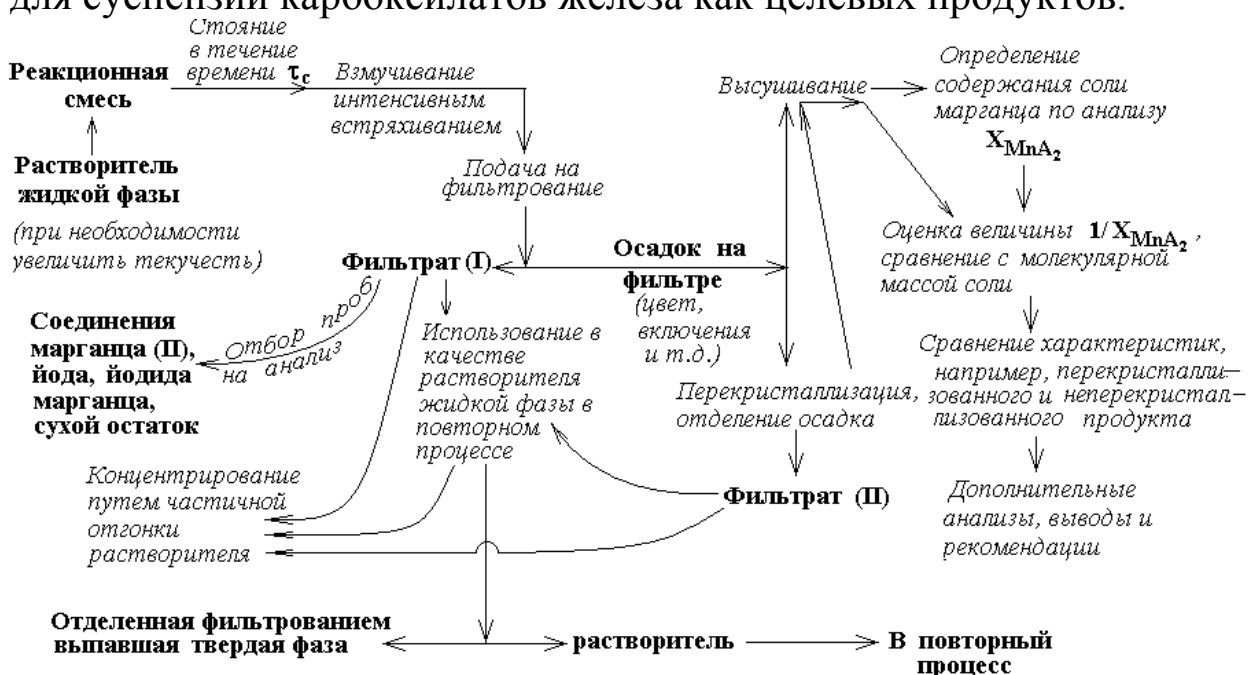
Рисунок 2- Вариант пооперационной схемы разделения реакционной смеси в виде суспензии продукта в жидкой фазе системы
