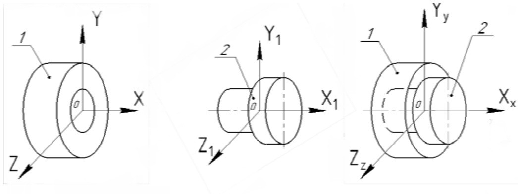
Рис.3. схема координатных систем двух сопрягаемых деталей:
