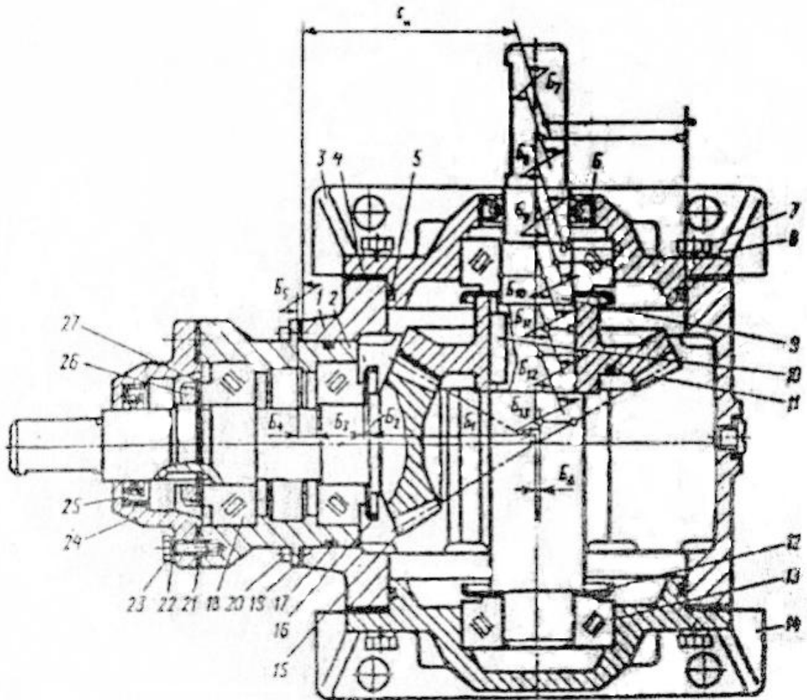
Рис.5. Конический редуктор
