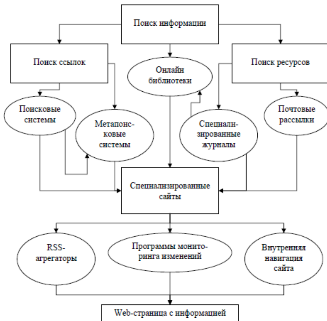
Рисунок 1. Схема поиска информации в WWW
