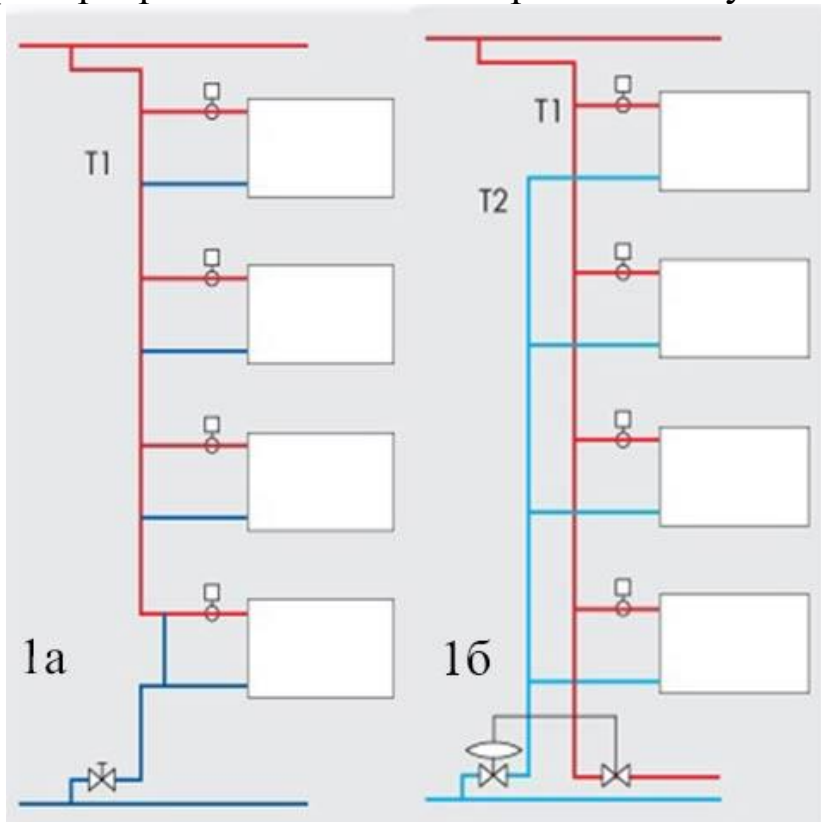
Рис.5 - Вертикальная система отопления
