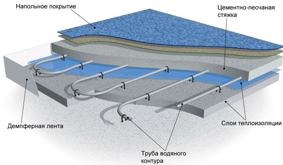
Рис.14 – Отопительная панель
