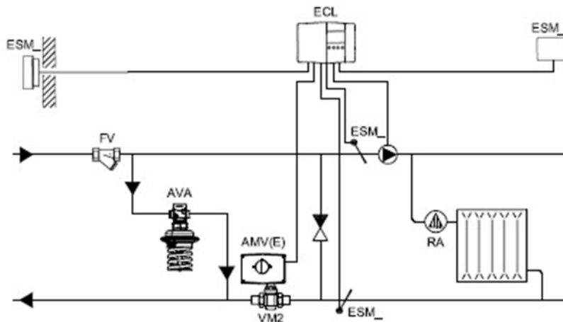
Рис.3 – Зависимая система отопления
