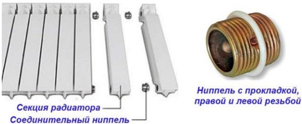
Рис.17 – Радиатор секционный
