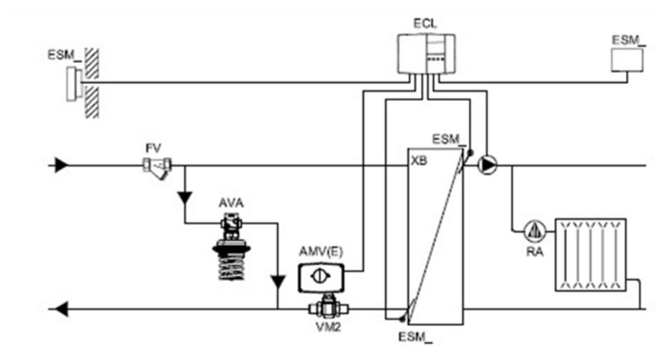
Рис.4– Независимая система отопления
