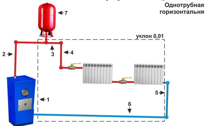
Рис.1 – Система отопления с естественной циркуляцией: 1- котел; 2- главный стояк; 3 – распределительная магистраль; 4, 5 – стояки; 6 – сборная магистраль
