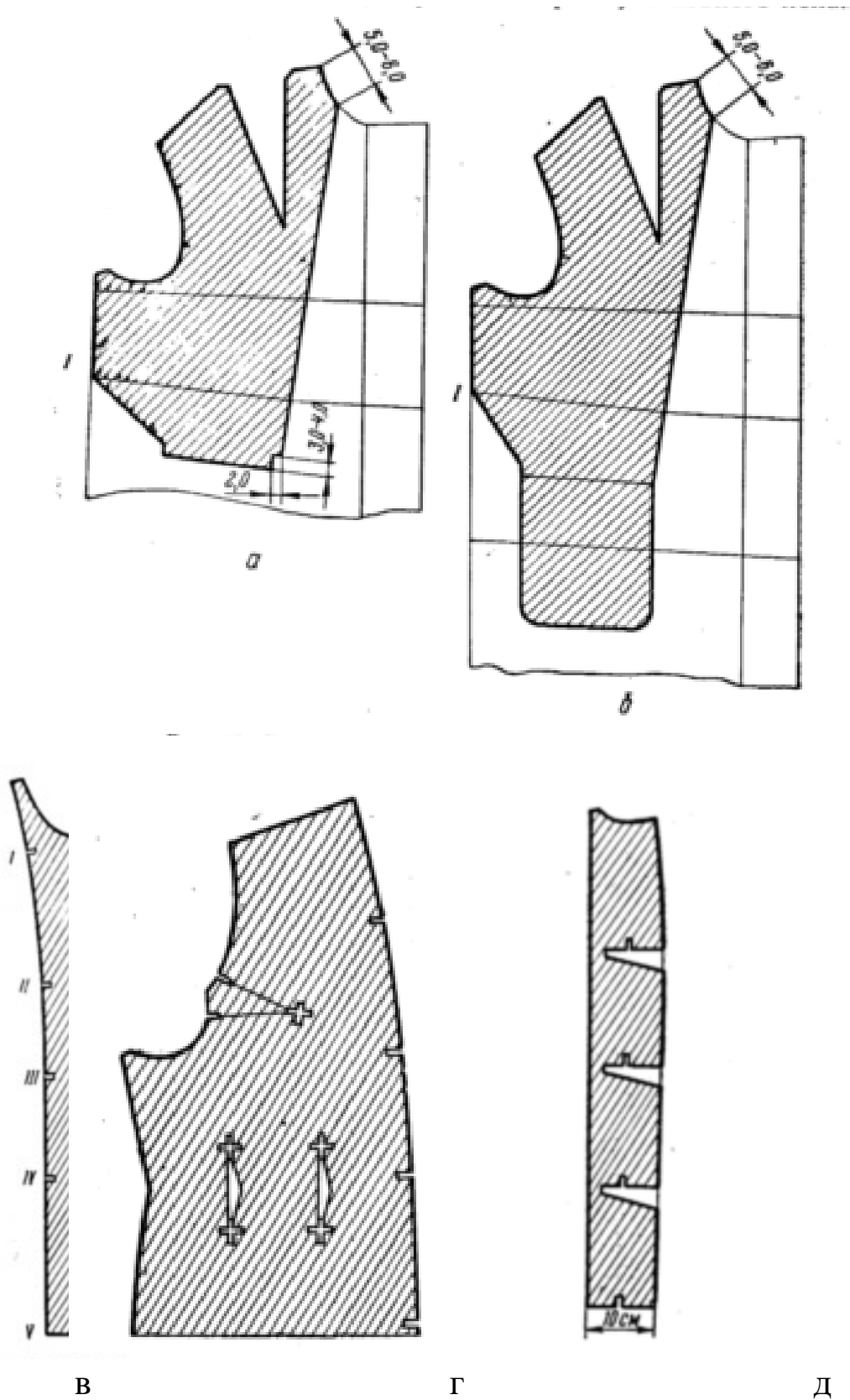
Рисунок Б2 - Схема построения вспомогательных лекал женской одежды для наметки: боковых прорезных карманов (рис.а), накладных карманов (рис.б), расположения надсечек на подборте (рис.в), вытачек и надсечек на подкладке (рис.г), петель на борте (рис.д)
