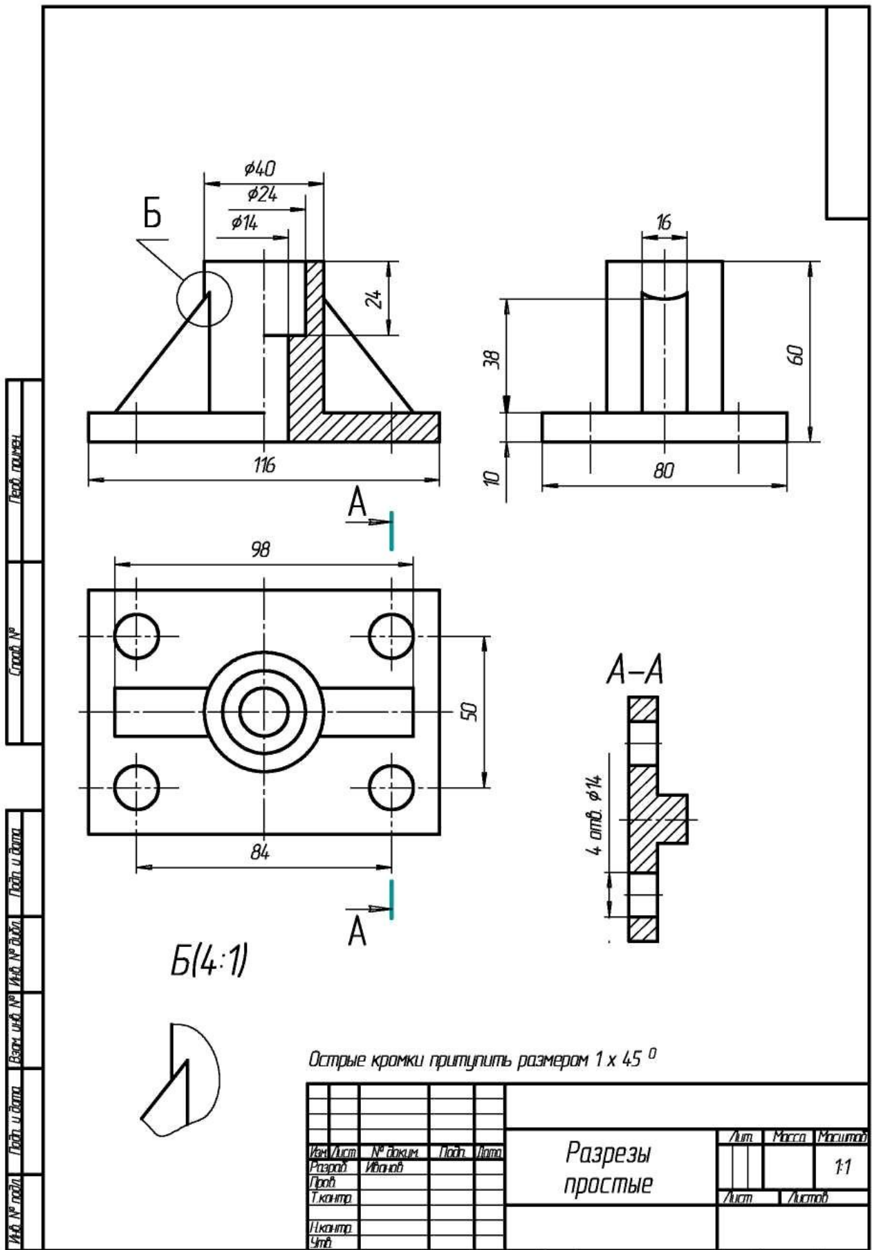
Рис. 3.22. - Пример выполнения задания «Разрезы»
