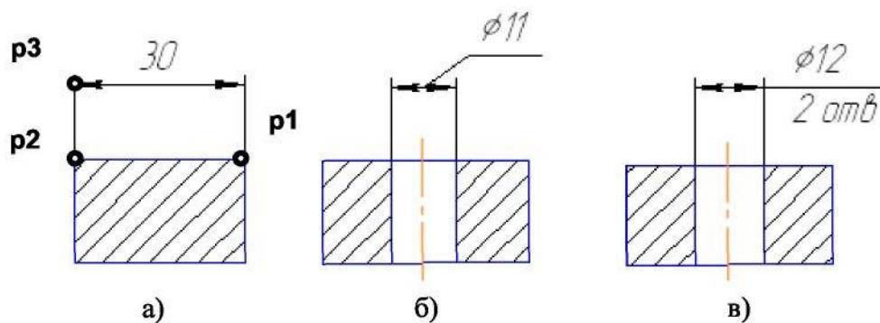
Рис. 2.8. - Варианты нанесения линейных размеров
