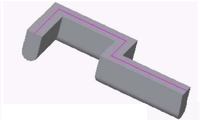
Рис. 5.32. - Формирование выреза по заданной траектории с использованием булевой операции Пересечение и булевой операции Вычитание элемента Рис. 5.33. - Формирование модели по заданной траектории с использованием булевой операции Пересечение и булевой операции Вычитание элемента
