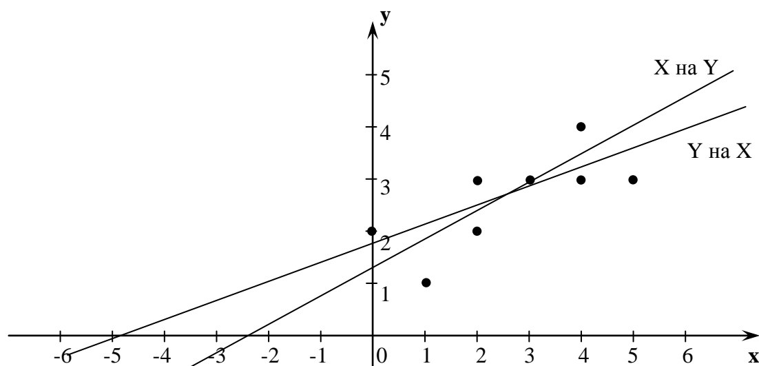
Рис. 3.1. Прямые регрессии
