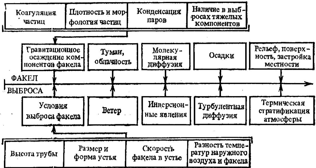
Рисунок 1 - Схема факторов, влияющих на рассеивание выбросов
