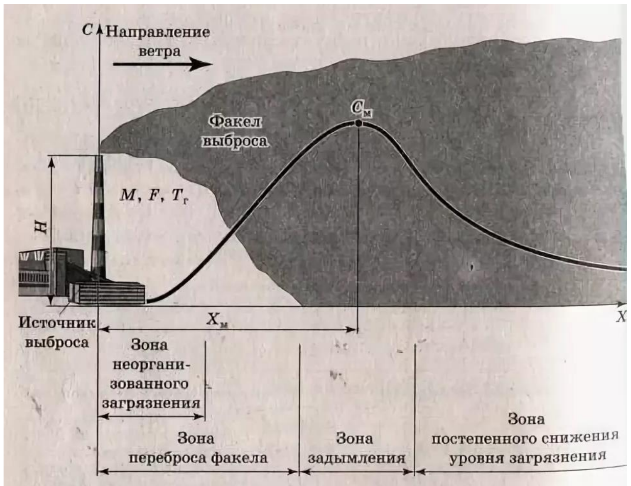
Рисунок 2 - Схема факторов, влияющих на рассеивание выбросов
