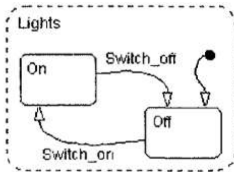
Рис. 6. Установка начального состояния
