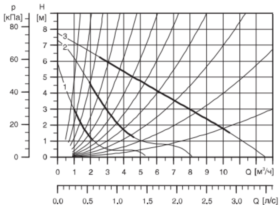
Рис.П.4.16. Характеристики регулируемого электронасоса UPS 40-80F
