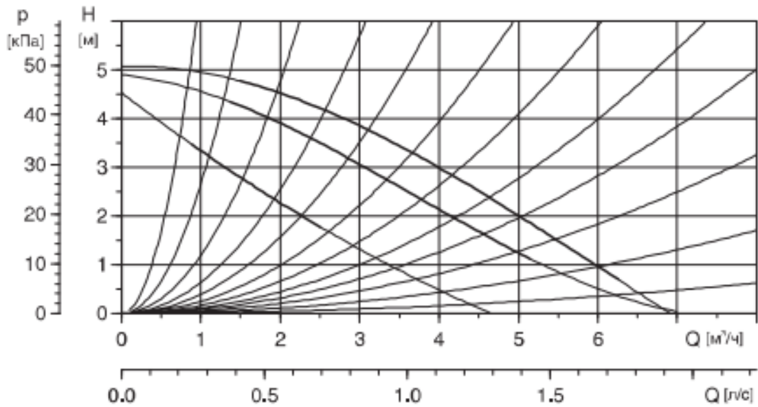
Рис.П. 4.7. Характеристики регулируемого электронасоса UPS 25-55
