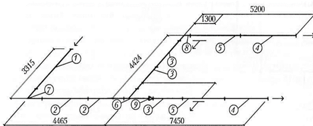
Рис. 2.5 - Фрагмент монтажной схемы системы вентиляции: 1,2,3 – прямые участки; 4 – прямой участок с торцевой сеткой; 5 – прямой участок с сеткой и движком; 6 – прямой участок с врезкой; 7, 8 – отводы; 9 – переход
