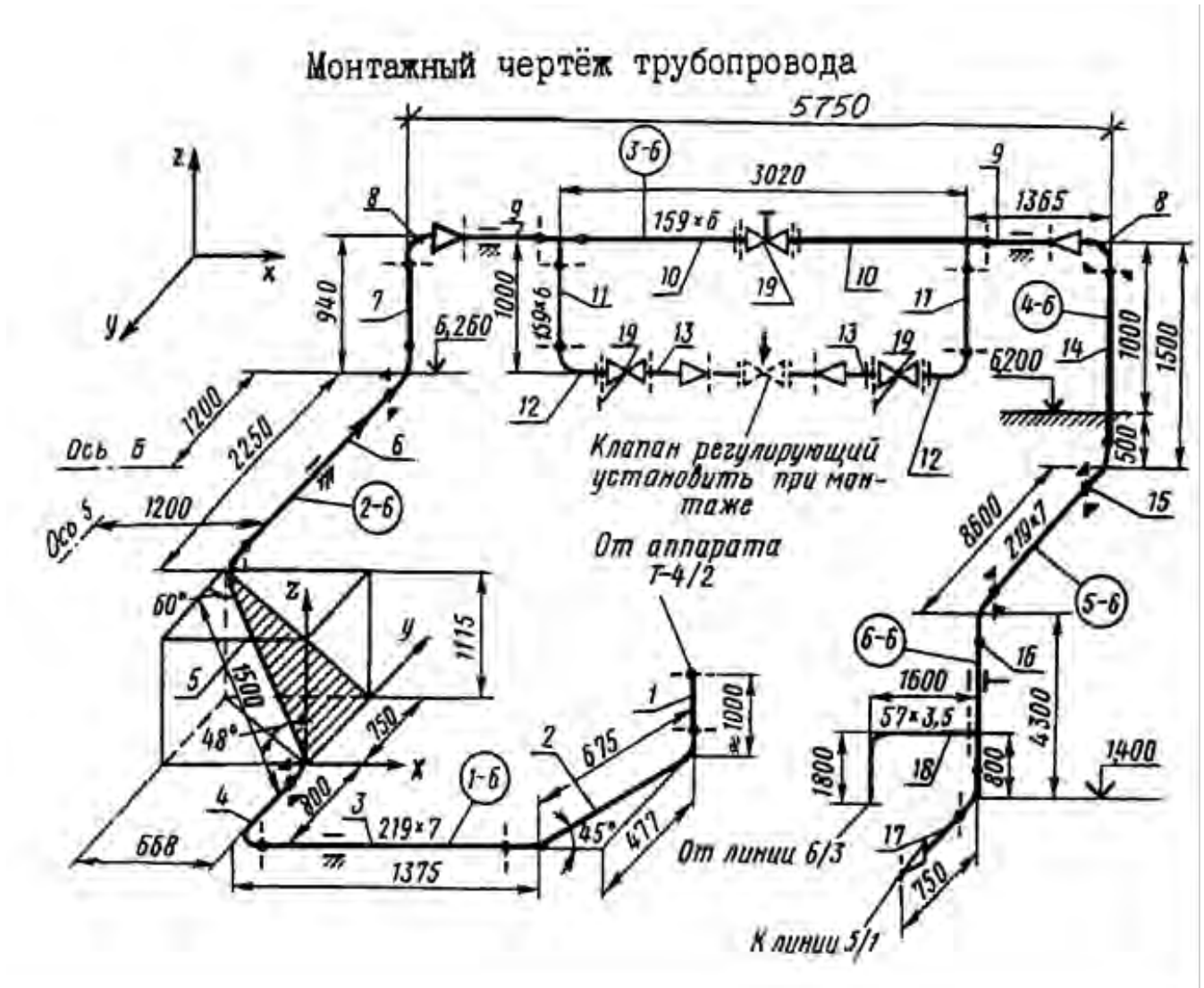
Рис 2.3 – Монтажный чертёж трубопровода
