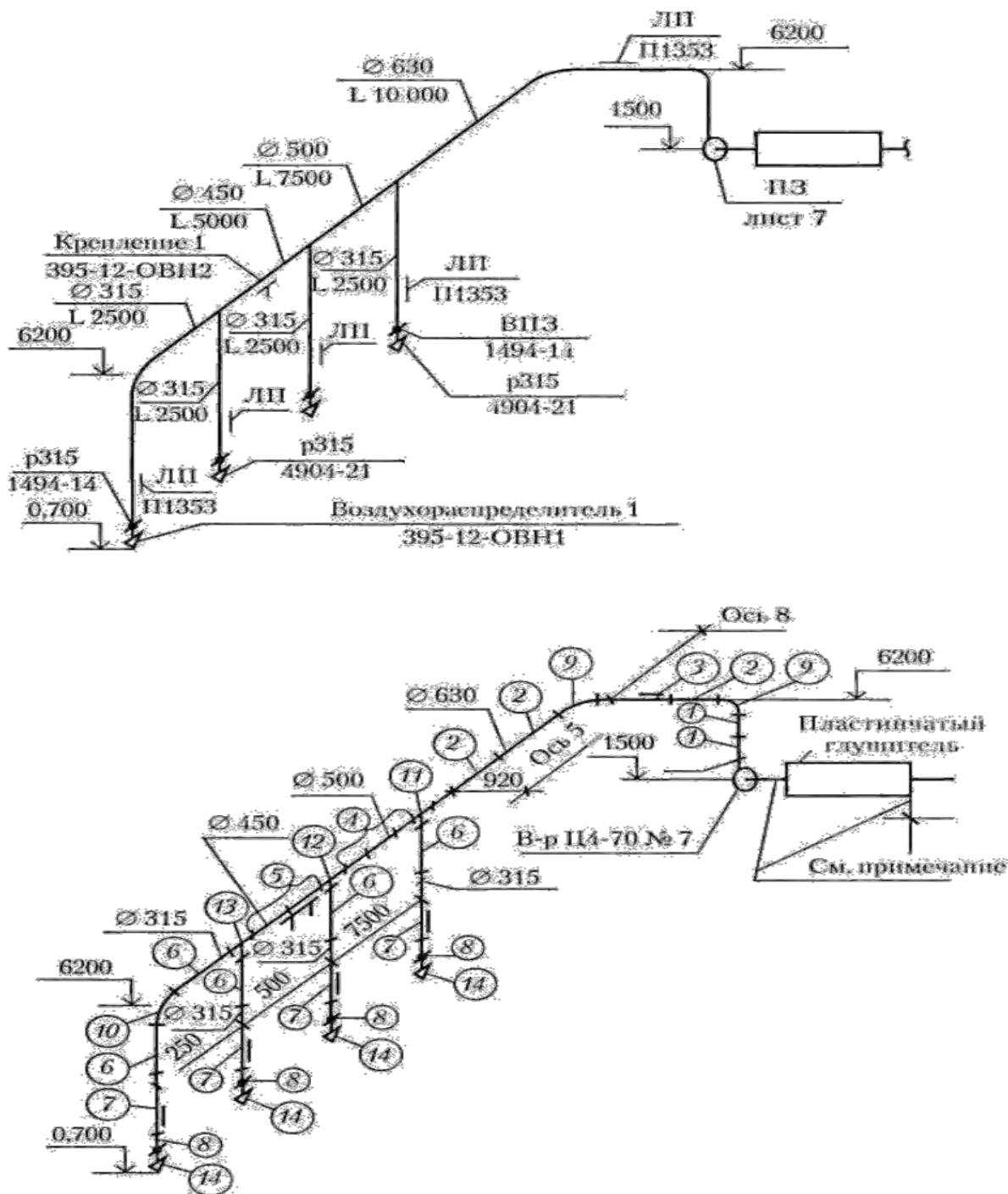
Рис. 2.4 - Аксонометрические схемы систем вентиляции: а – схема рабочего чертежа; б – монтажная схема; 1 – 14 – унифицированные детали
