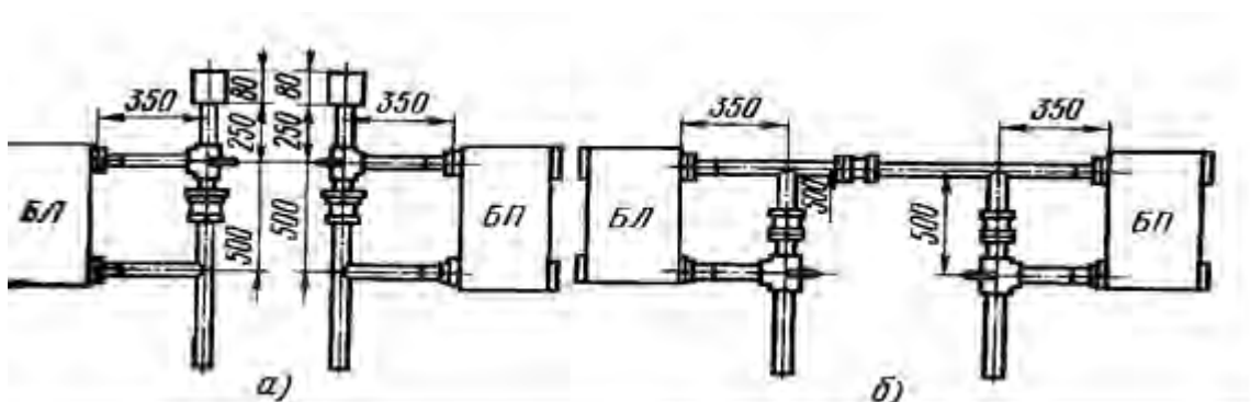
Рис.2.2 - Радиаторные правый (БП) и левый (БЛ) блоки для систем с трёхходовыми кранами: а – для первого и промежуточного этажей; б – для верхнего этажа.
