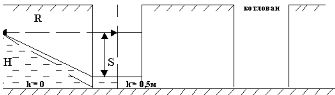
Рис. 5. Перехват потока грунтовых вод канавой
