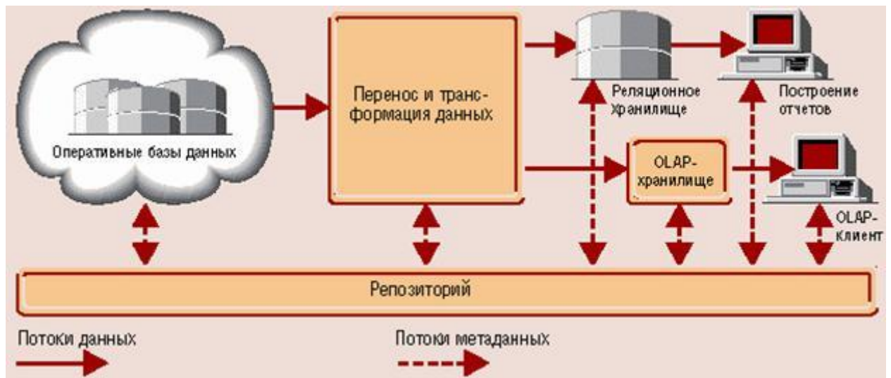
Рисунок 1. Место OLAP в информационной структуре предприятия
