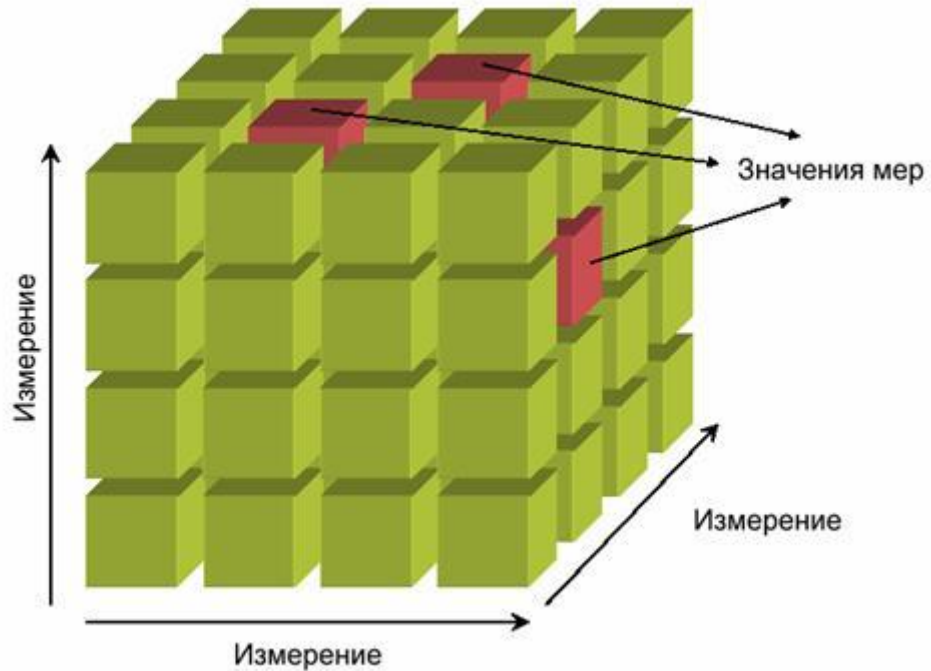
Рисунок 1. OLAP – куб (гиперкуб, метакуб)
