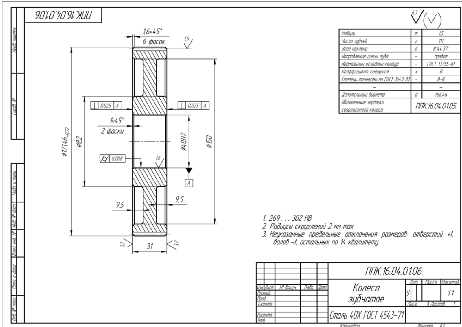
Рисунок 6.2 – Рабочий чертеж зубчатого колеса
