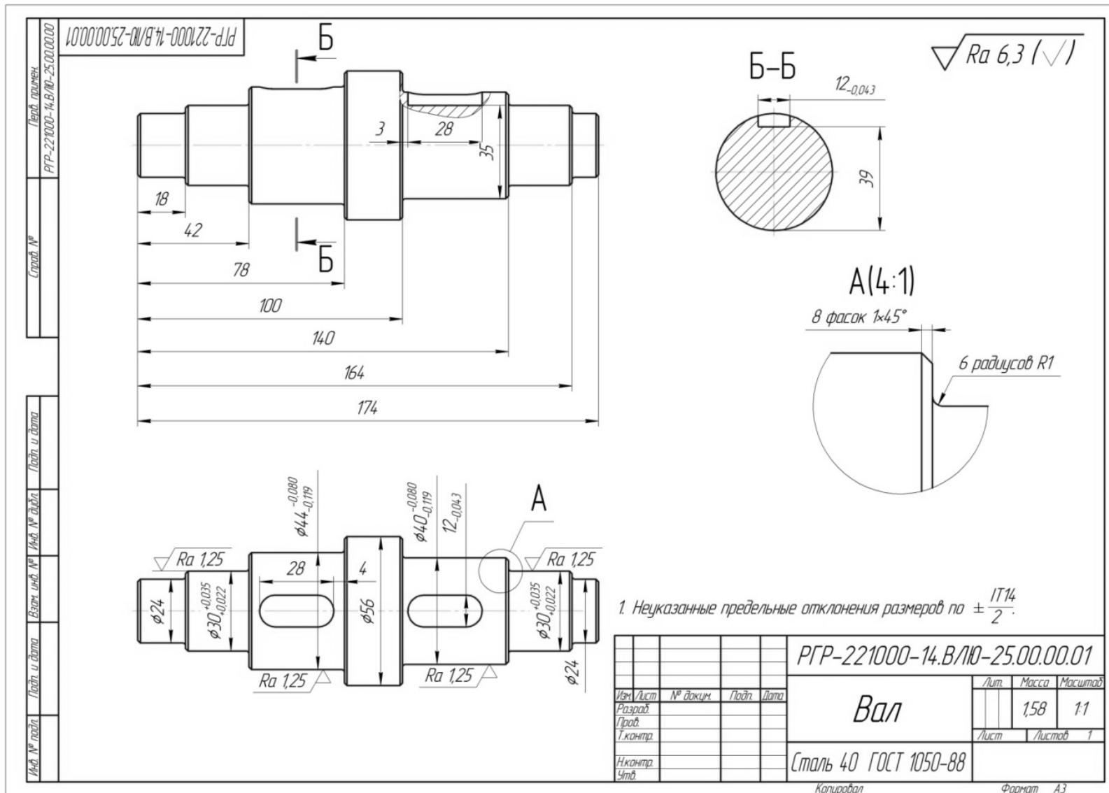
Рисунок 6.1 – Рабочий чертеж вала
