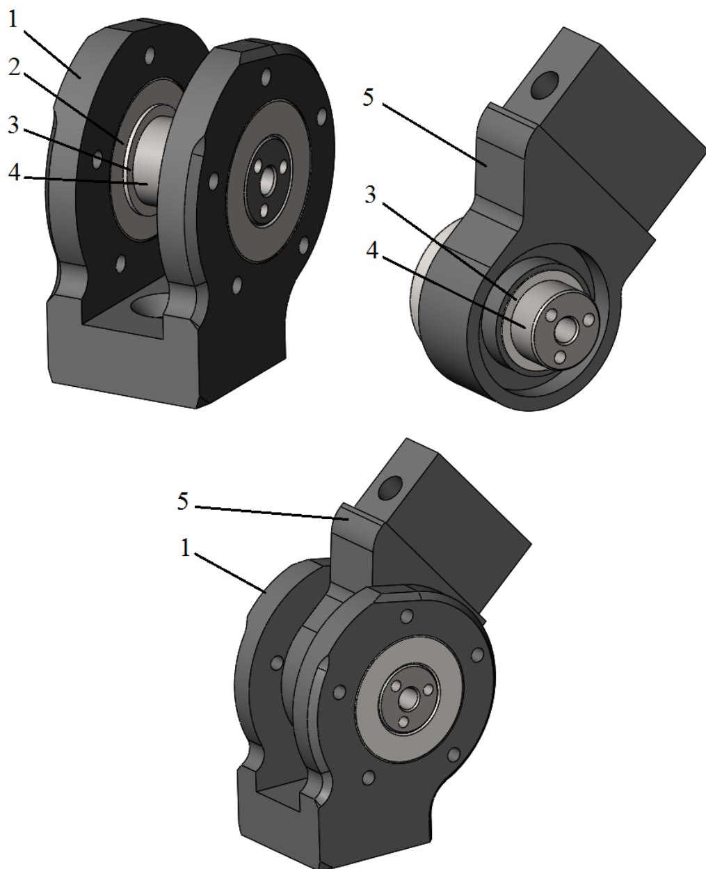
Рисунок 4.3 – Трехмерная модель однокоординатного шарнира: 1 – вилка; 2 – подшипник; 3 – шайба; 4 – ось; 5 – проушина звена
