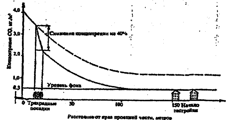
Рисунок 2 - Снижение концентрации CO за счет устройств трехрядных посадок деревьев.
