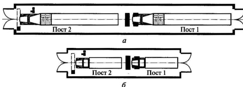
Рис. 4.8. Типовые планировочные решения П/П «МГСТК» для линий проверки грузовых автомобилей и автобусов:
