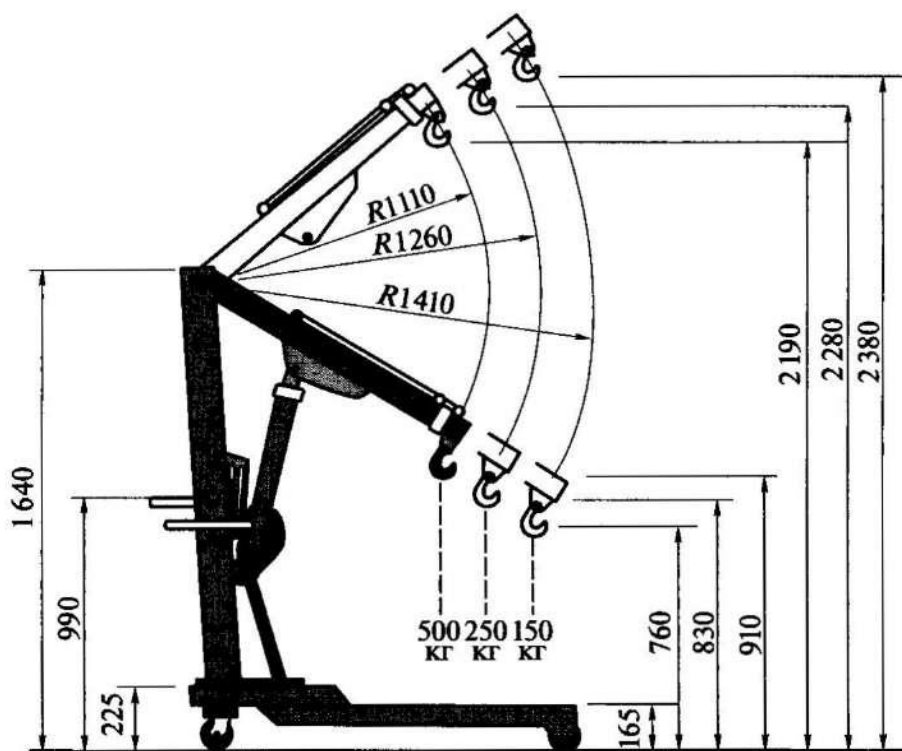
Рис. 5.15. Передвижной кран
