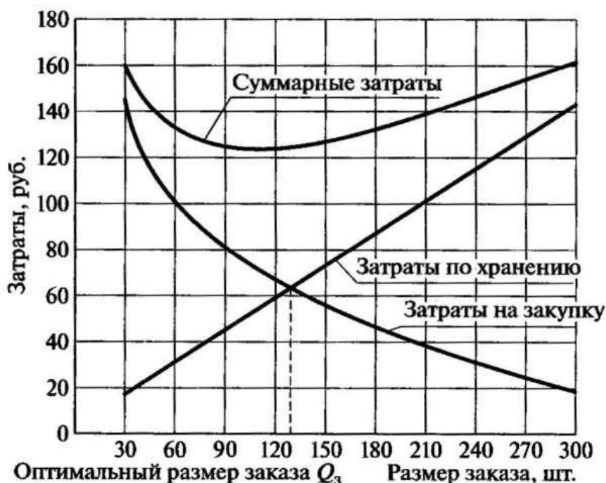
Рис. 9.4. График для определения оптимального размера заказа запчастей
