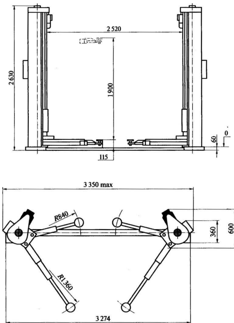
Рис. 5.10. Двухстоечный электромеханический подъемник
