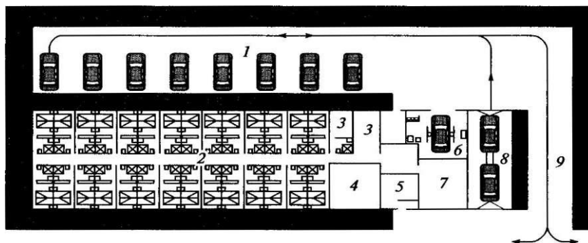
Рис. 4.13. Планировка мотеля:
