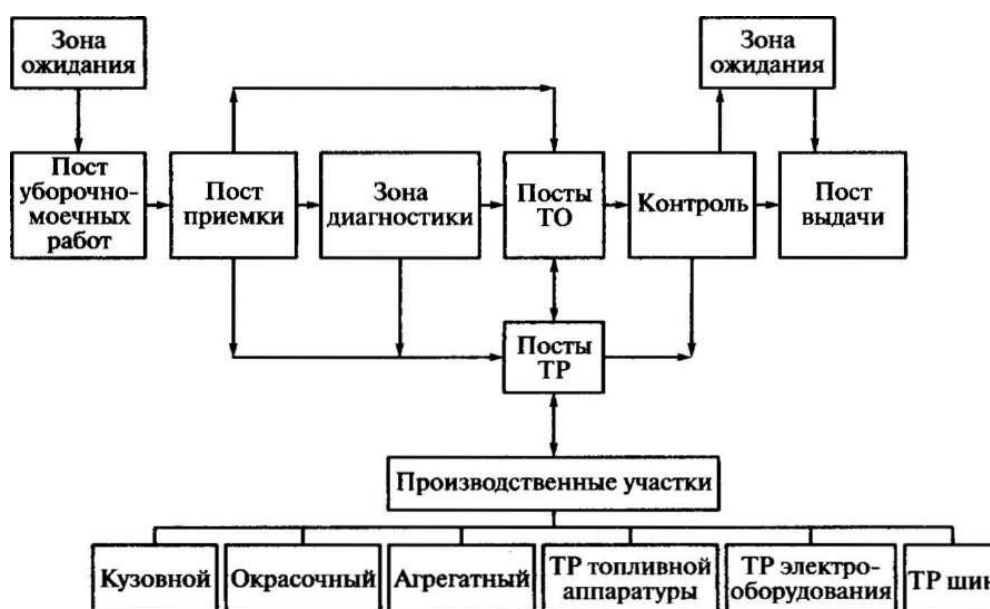
Рис. 7.2. Функциональная схема СТОА
