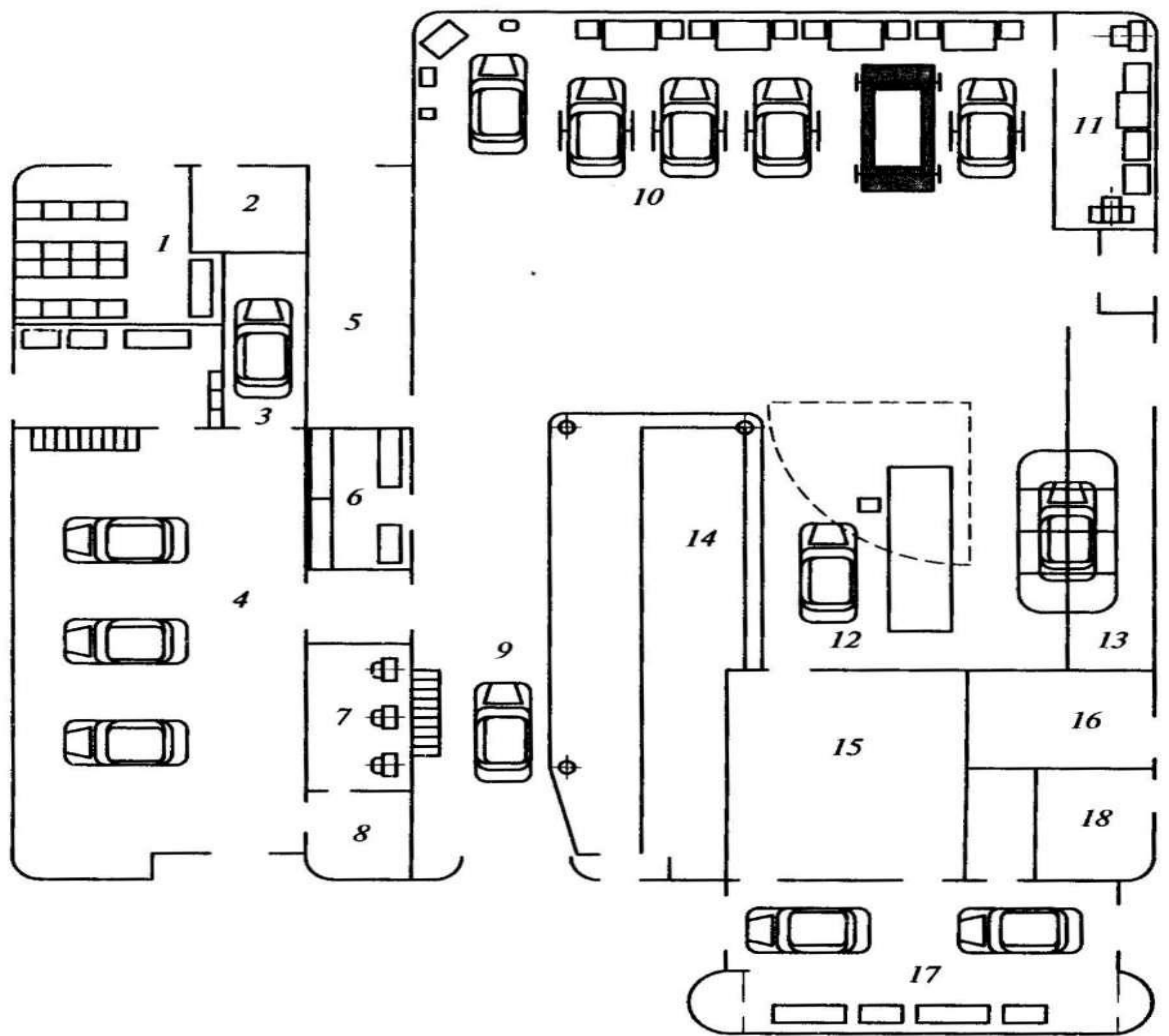
Рис. 4.3. Планировка станции технического обслуживания на 15 рабочих постах: 1 — склад запасных частей, агрегатов и материалов; 2 — теплогенераторная; 3 — окрасочно-сушильная камера; 4 — участок подготовки автомобилей к окраске; 5 — кладовая масел и смазочных материалов; 6 — промкладовая; 7 — компрессорная; 8 — тамбур-шлюз; 9 — пост приемки-выдачи; 10 — посты ТО и ТР; 11 — шиномонтажный участок; 12 — посты сварки и жестяницких работ; 13 — пост правки и растяжки кузовов; 14 — клиентская, пункт обмена вал ют, кабинеты сотрудников СТО; 15 — бытовые помещения; 16 — электрощитовая; 17 — участок мойки автомобилей; 18 — индивидуальный тепловой пункт
