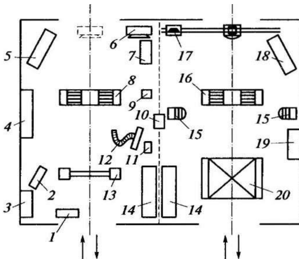
Рис. 7.4. Планировка двухпостового участка диагностирования на СТОА: / — площадочный стенд для проверки установки управляемых колес; 2 — пульт управления площадочного стенда; 3 — инструментальный шкаф; 4 — стеллаж с комплектом СТД углубленного диагностирования; 5 — пульт управления и индикации тягового стенда; 6 — вентилятор; 7— мотор-тестер; 8 — роликовый узел тягового стенда; 9 — расходомер топлива; 10— воздухоподдаточная колонка; 11 — газоанализатор; 12 — устройство для отвода отработавших газов; 13 — стенд для проверки амортизаторов; 14 — верстак; 15 — станок для балансировки колес на автомобиле; 16 — роликовый узел тормозного стенда; 17 — прибор для проверки установки фар; 18— пульт управления и индикации тормозного стенда; 19— верстак; 20— подъемник
