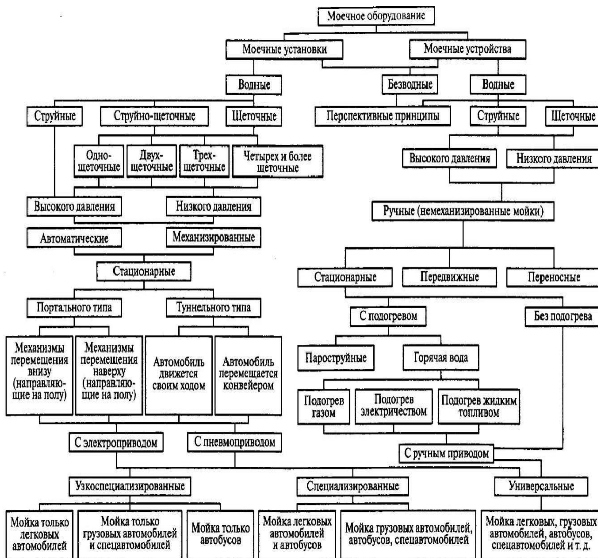
Рис. 5.3. Классификация оборудования для мойки подвижного состава автомобильного транспорта
