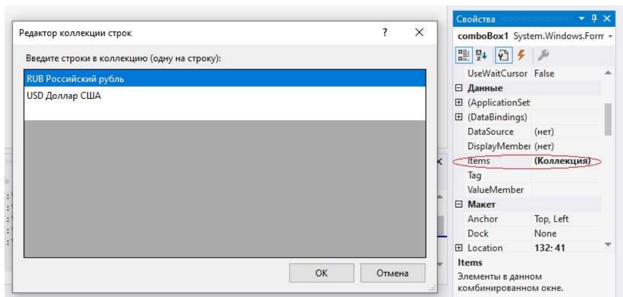
Рисунок 4 – Добавление элементов в раскрывающийся (выпадающий) список
